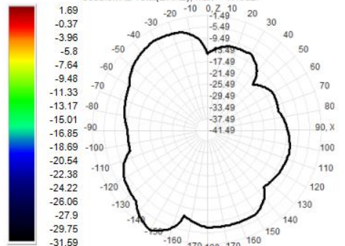
5850.0MHz Total(E1-XZ), Max= -1.49dBi
