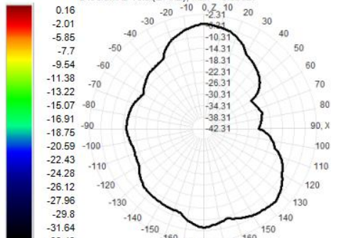
5850.0MHz Total(E1-XZ), Max= -1.49dBi
