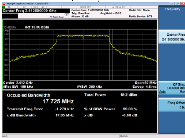
802.11n(HT20) 2412MHz
