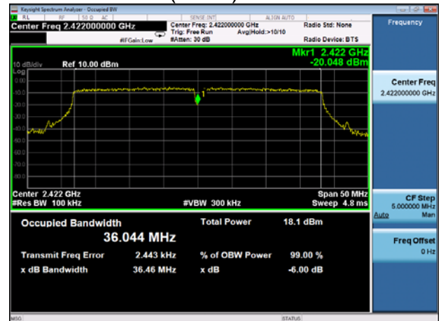
802.11n(HT40) 2422MHz
