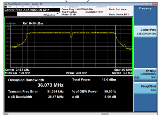
802.11n(HT40) 2452MHz
