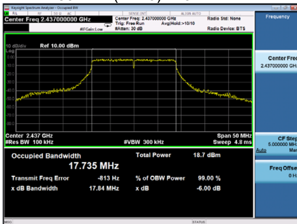
802.11n(HT20) 2437MHz
