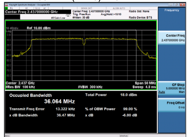
802.11n(HT40) 2437MHz
