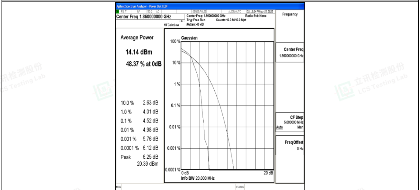
Band2-20MHz-16QAM-18700-1RB#0-PASS
