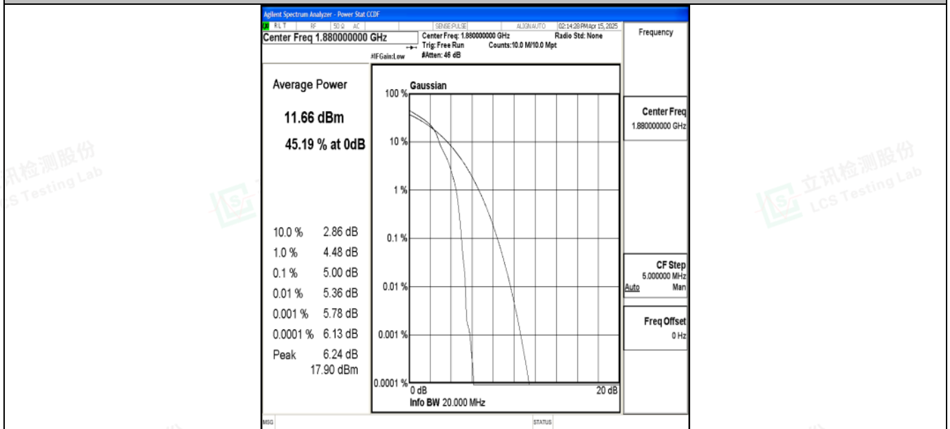
Band2-20MHz-16QAM-18900-1RB#0-PASS
