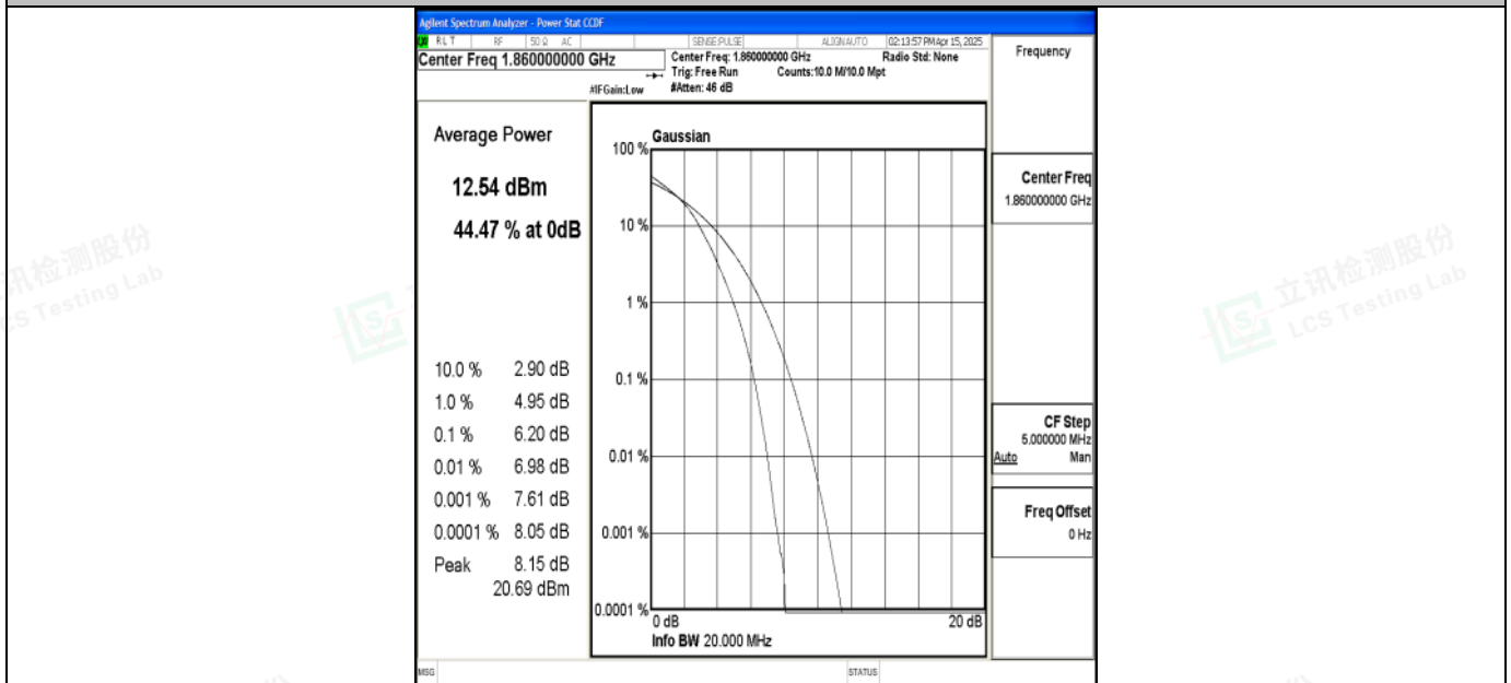
Band2-20MHz-16QAM-18700-100RB#0-PASS
