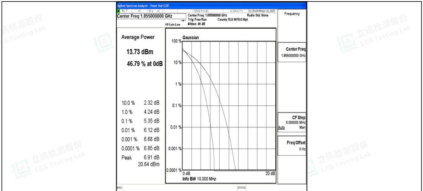
Band2-10MHz-QPSK-18650-50RB#0-PASS
