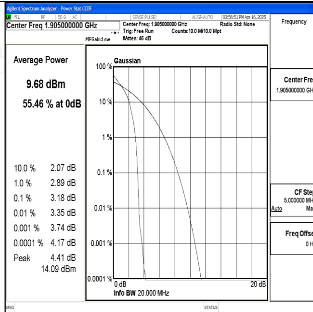
Band25-20MHz-QPSK-26590-1RB#0-PASS
