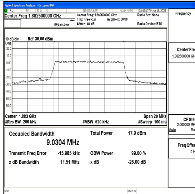
Band25-10MHz-QPSK-26365-50RB#0-PASS
