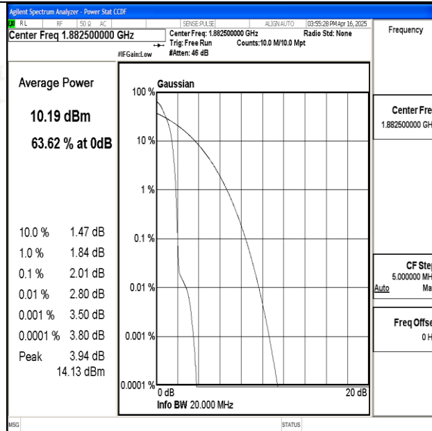
Band25-20MHz-QPSK-26365-1RB#0-PASS
