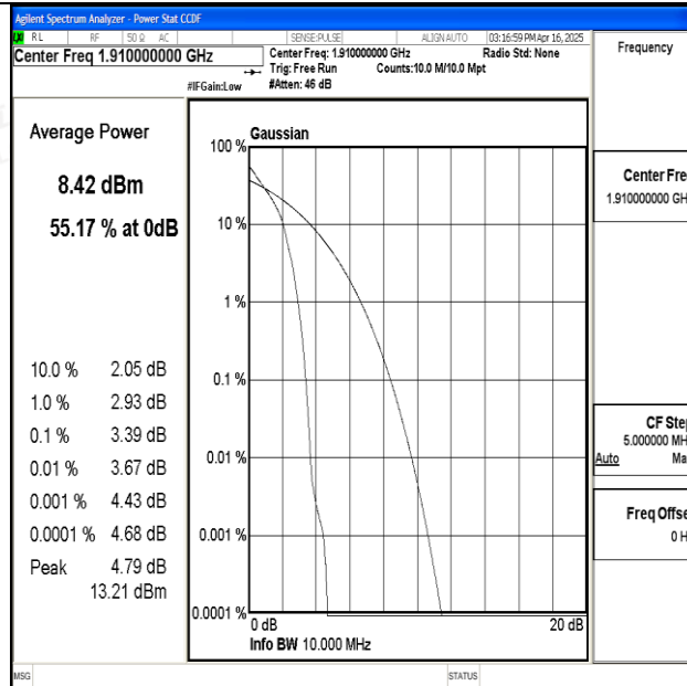
Band25-10MHz-QPSK-26640-1RB#0-PASS
