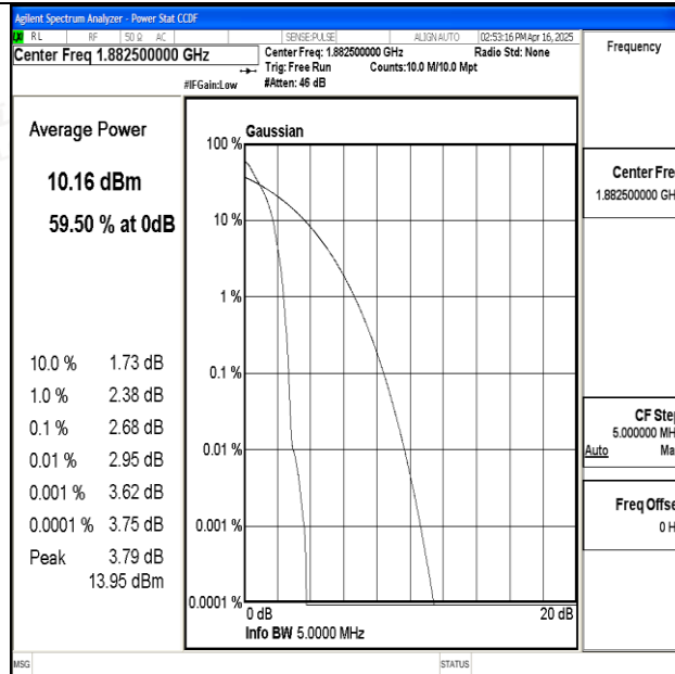
Band25-5MHz-QPSK-26365-1RB#0-PASS
