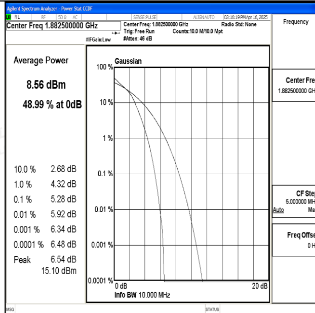
Band25-10MHz-16QAM-26365-50RB#0-PASS
