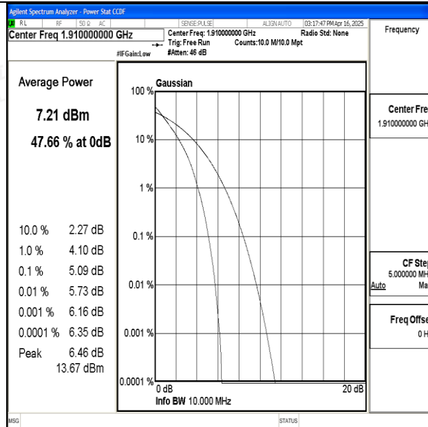
Band25-10MHz-QPSK-26640-50RB#0-PASS
