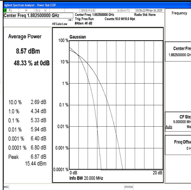
Band25-20MHz-16QAM-26365-100RB#0-PASS
