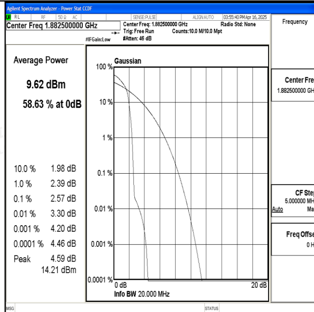
Band25-20MHz-16QAM-26365-1RB#0-PASS
