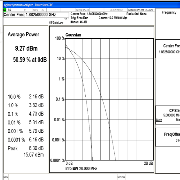
Band25-20MHz-QPSK-26365-100RB#0-PASS
