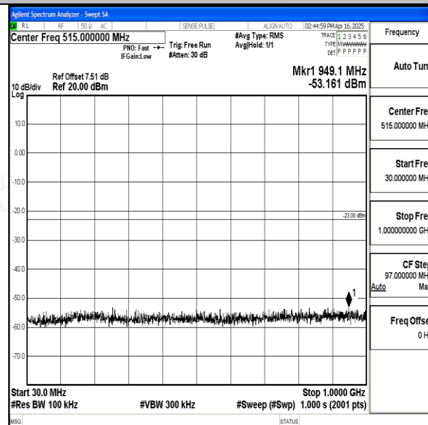
Band25 5MHz 16QAM 26065 1RB#0 30~1000 30~1000
