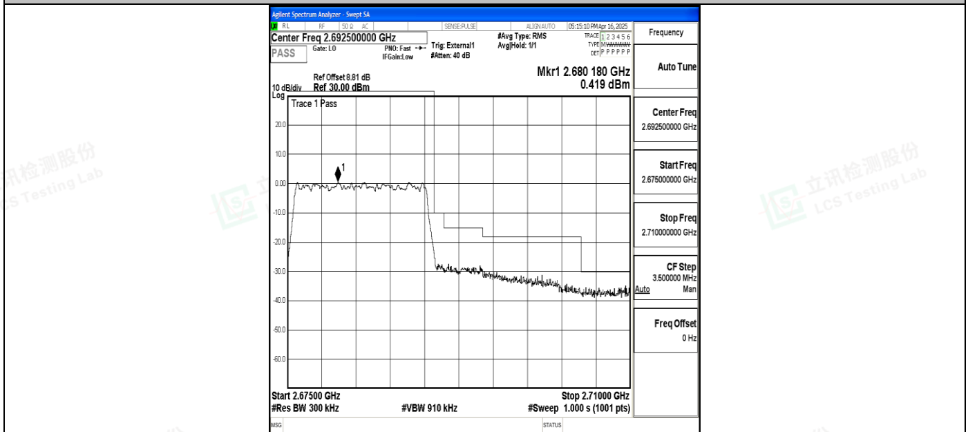
Band41_15MHz_QPSK_41515_75RB#0
