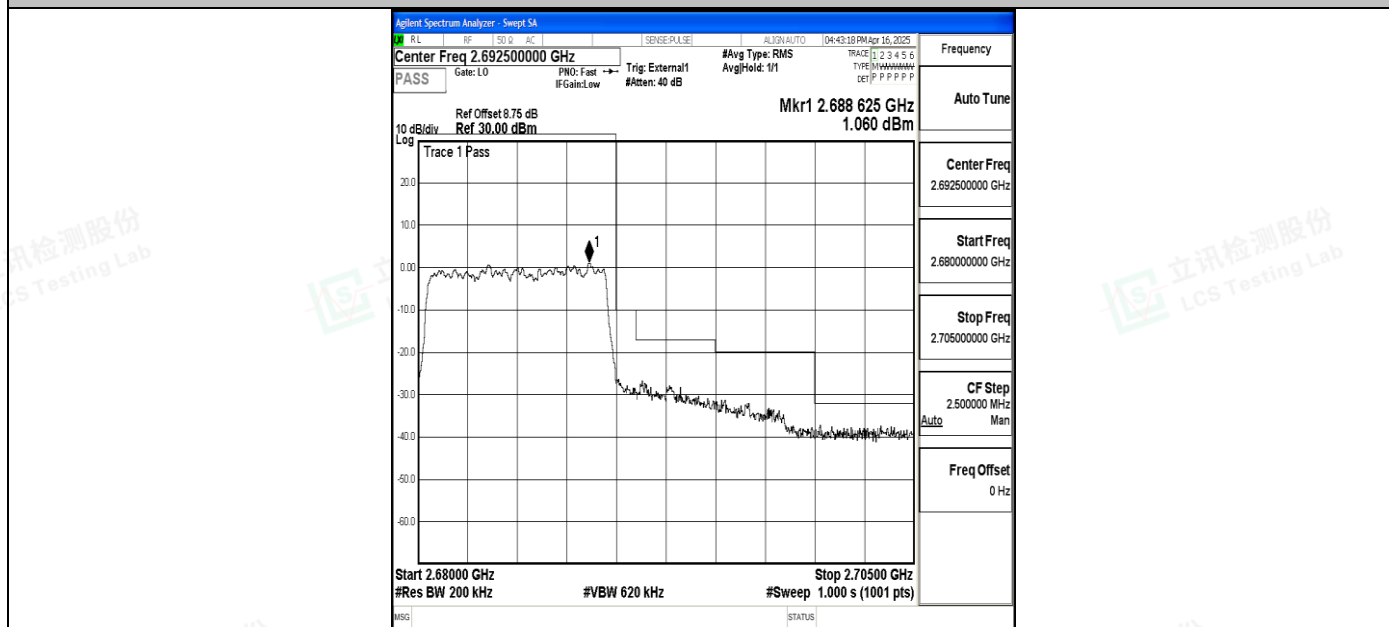
Band41_10MHz_QPSK_41540_50RB#0
