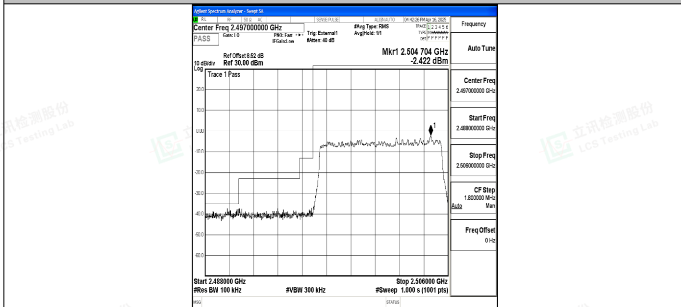
Band41_10MHz_QPSK_39700_50RB#0
