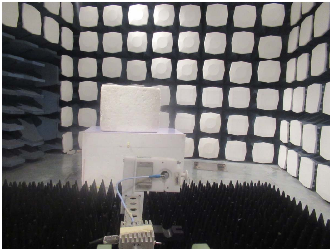
18GHz-26GHz
