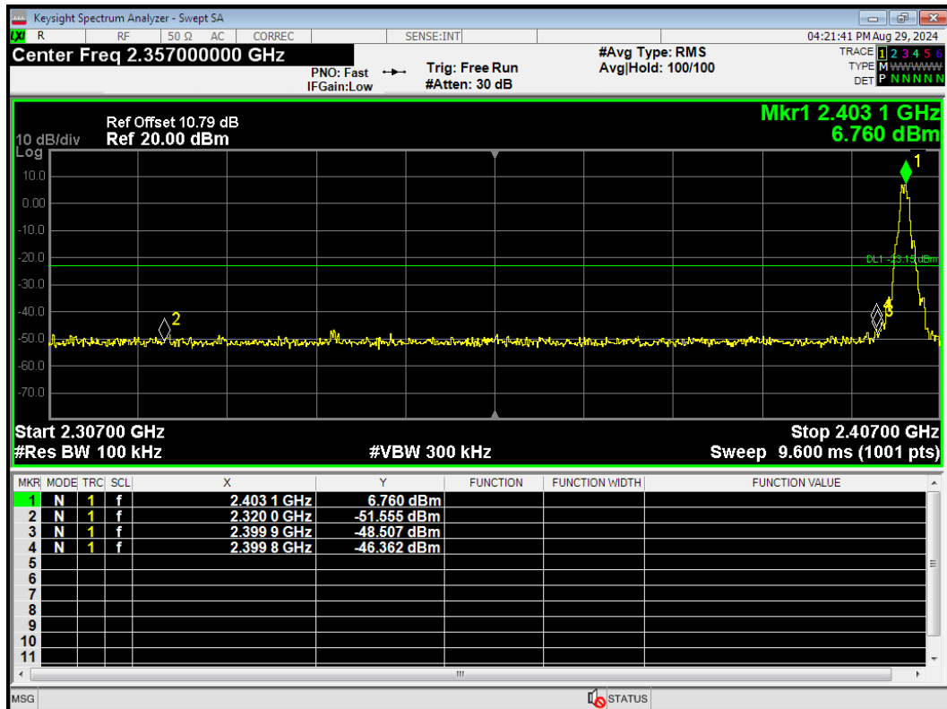
Band Edge 2403MHz Emission
