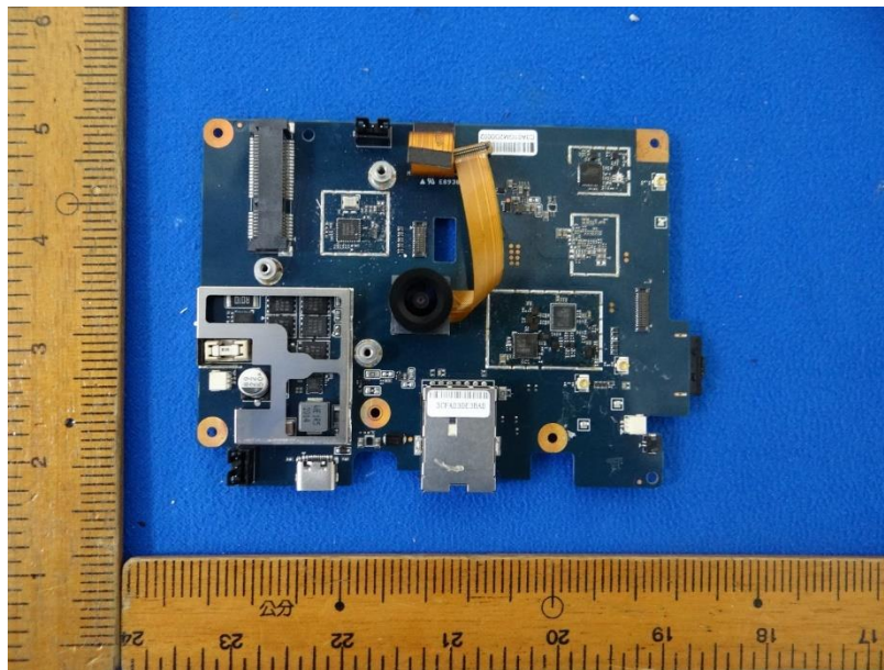
(6) EUT Photo
