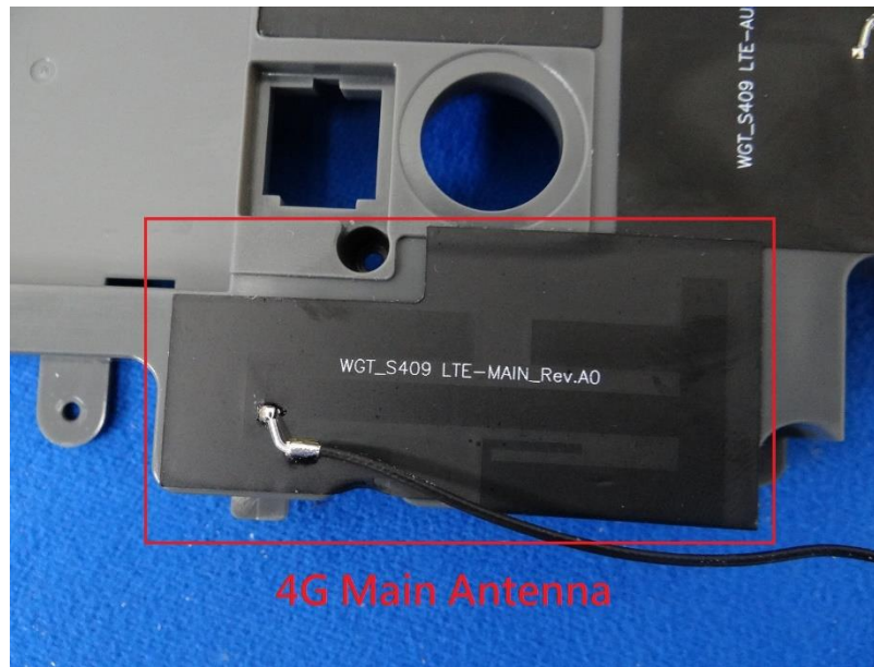
(13) EUT Photo
