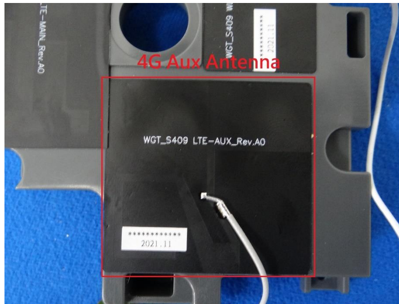
(15) EUT Photo
