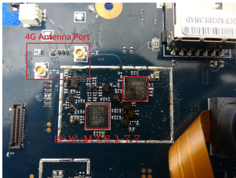
(8) EUT Photo
