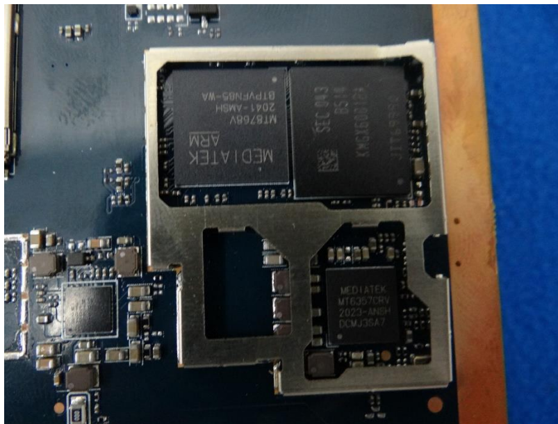
(12) EUT Photo
