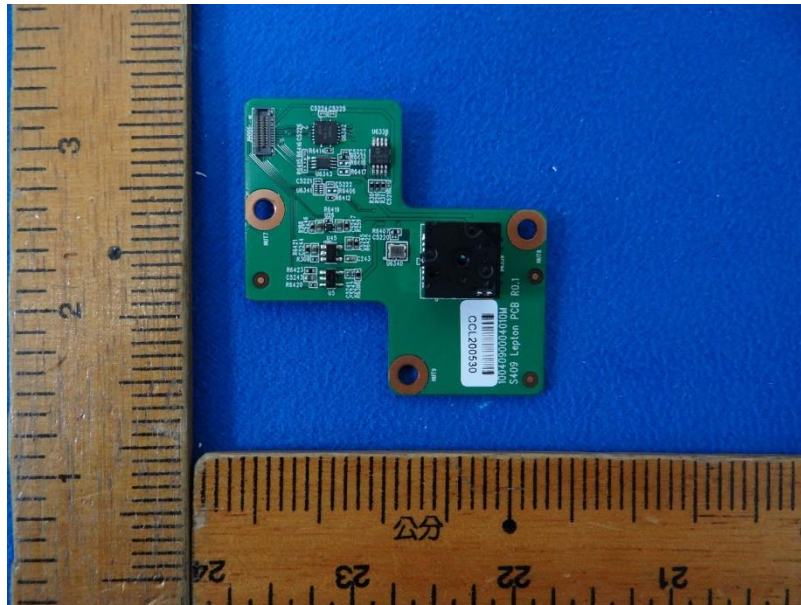
(4) EUT Photo
