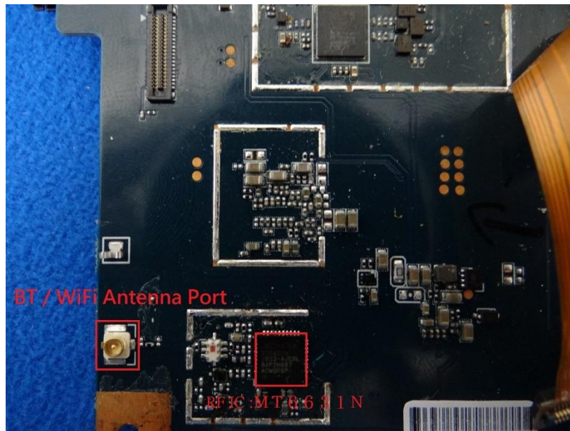
(9) EUT Photo
