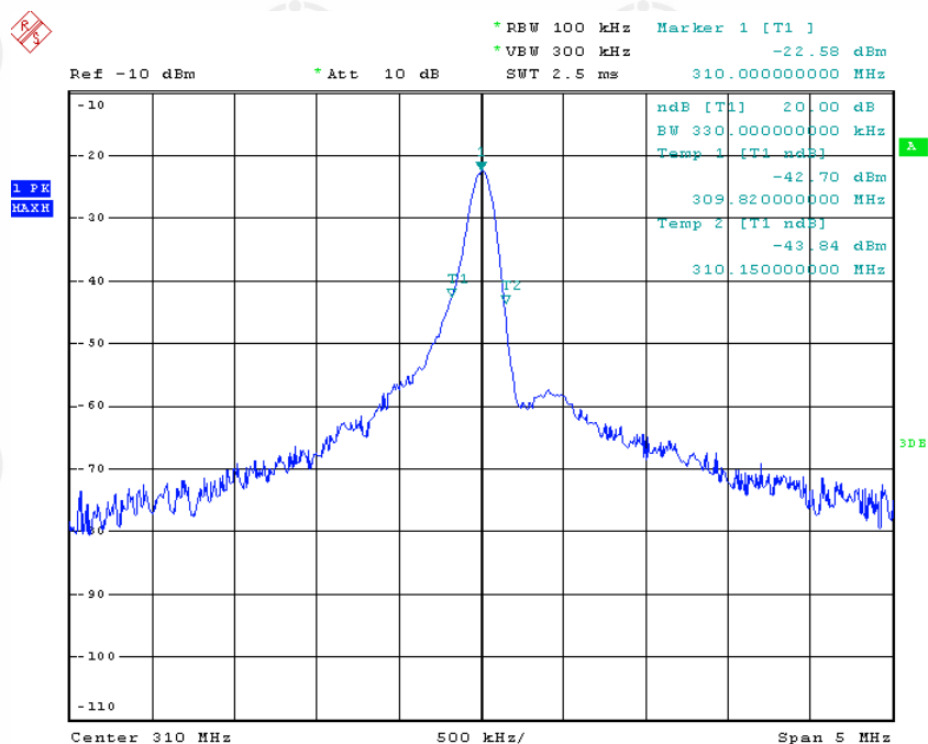
20dB BW
