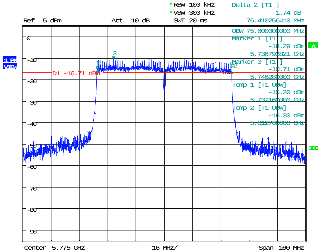
Plot 1. 18 802.11ac 80MHz, 5775MHz
