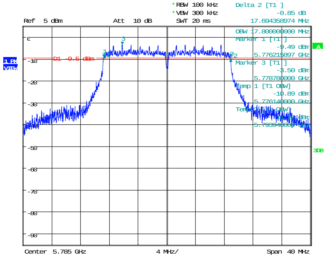
Plot 1. 14 802.11n 20MHz, 5785MHz
