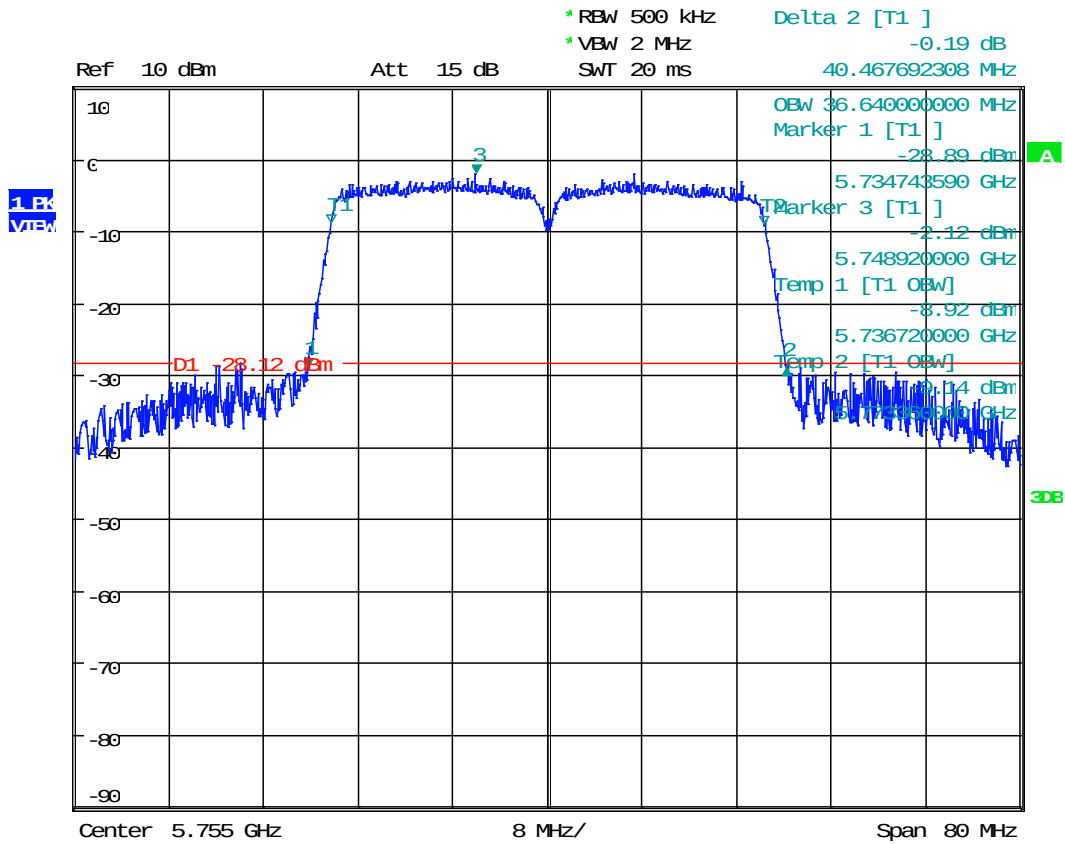
Plot 1.7 802.11n 40MHz, 5755MHz
