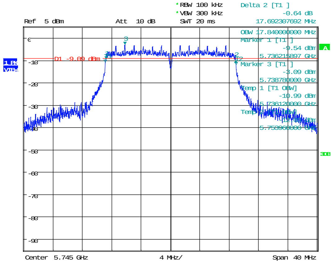
Plot 1. 13 802.11n 20MHz, 5745MHz
