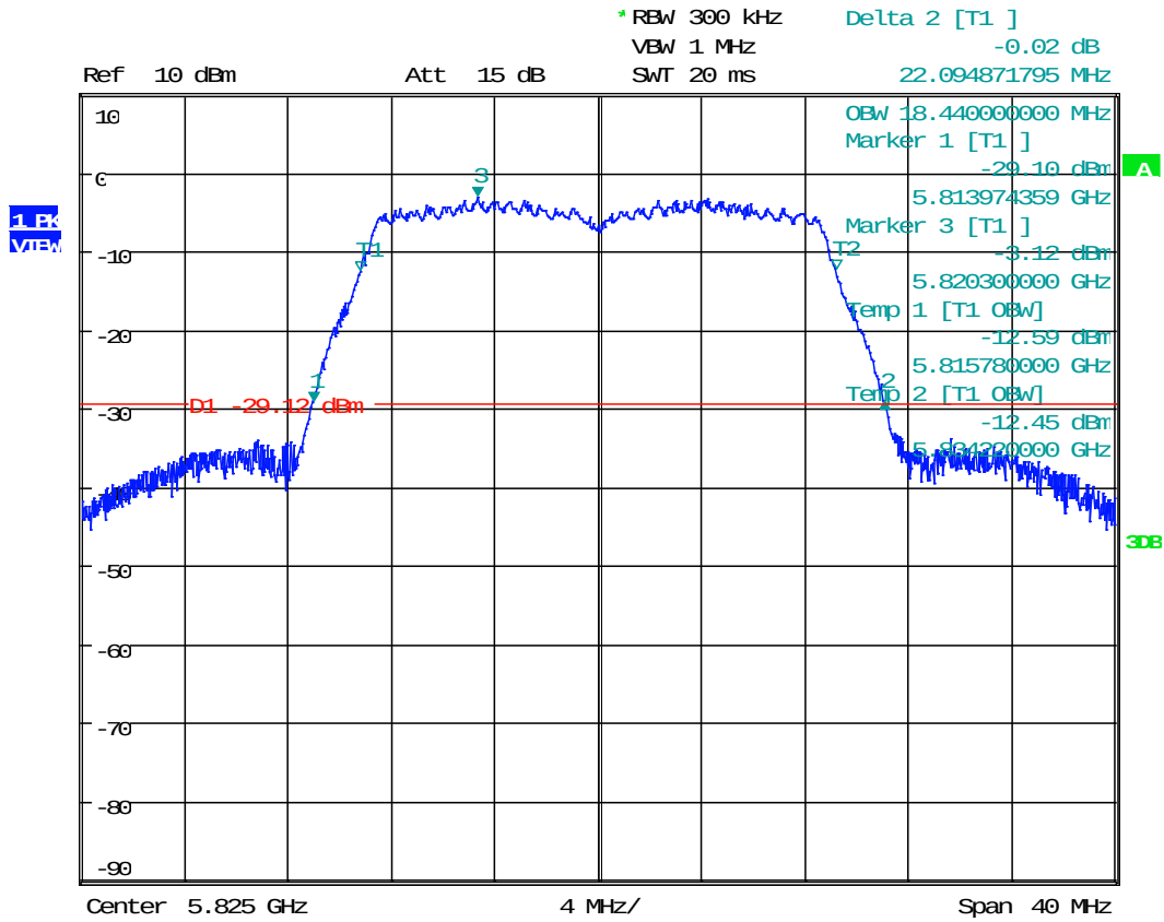
Plot 1. 6 802.11n 20MHz, 5825MHz
