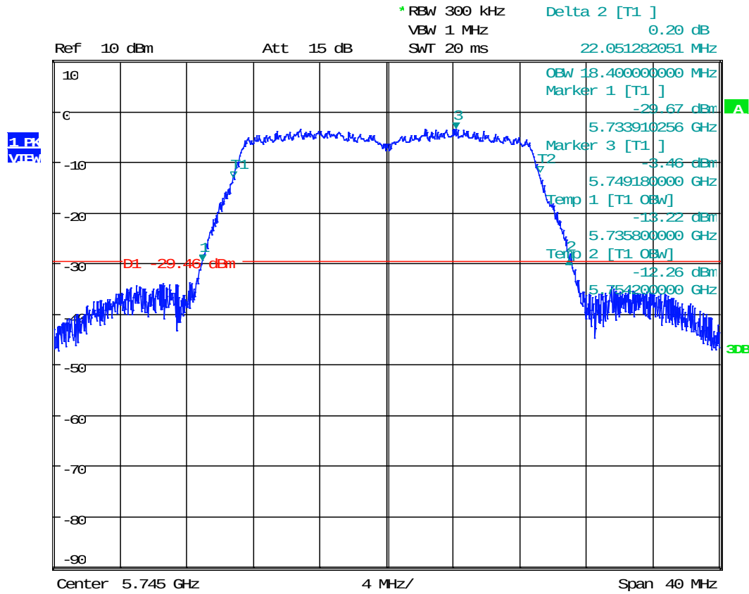
Plot 1. 4 802.11n 20MHz, 5745MHz
