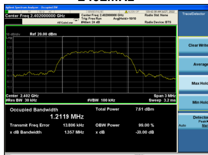
2402MHz
