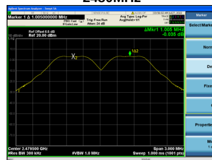
2480MHz
