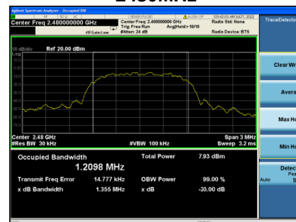
2480MHz
