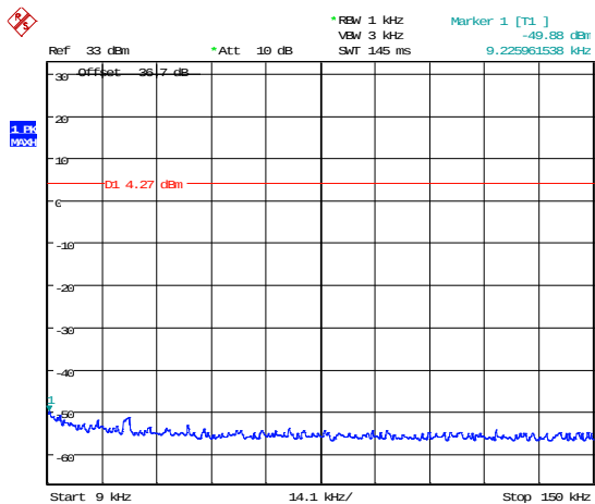
914.8MHz 9-150kHz
