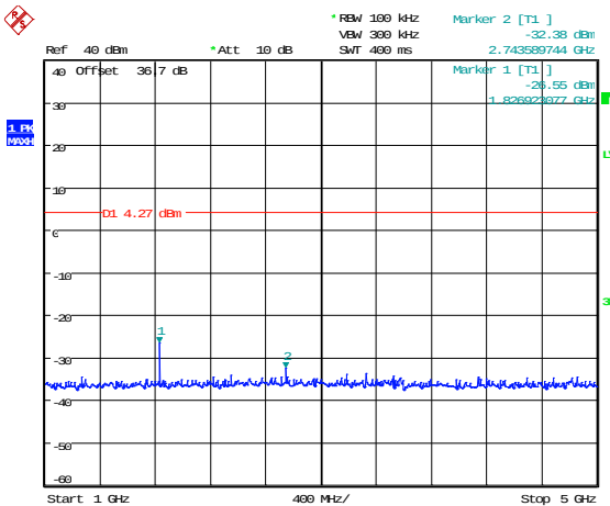
914.8MHz 1GHz-5GHz
