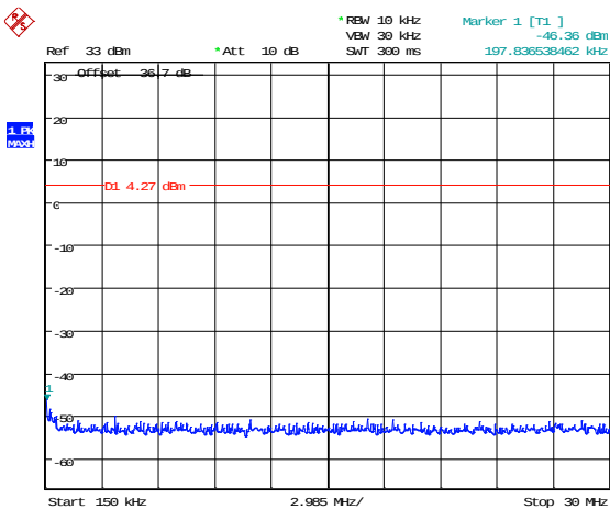
914.8MHz 150-30MHz
