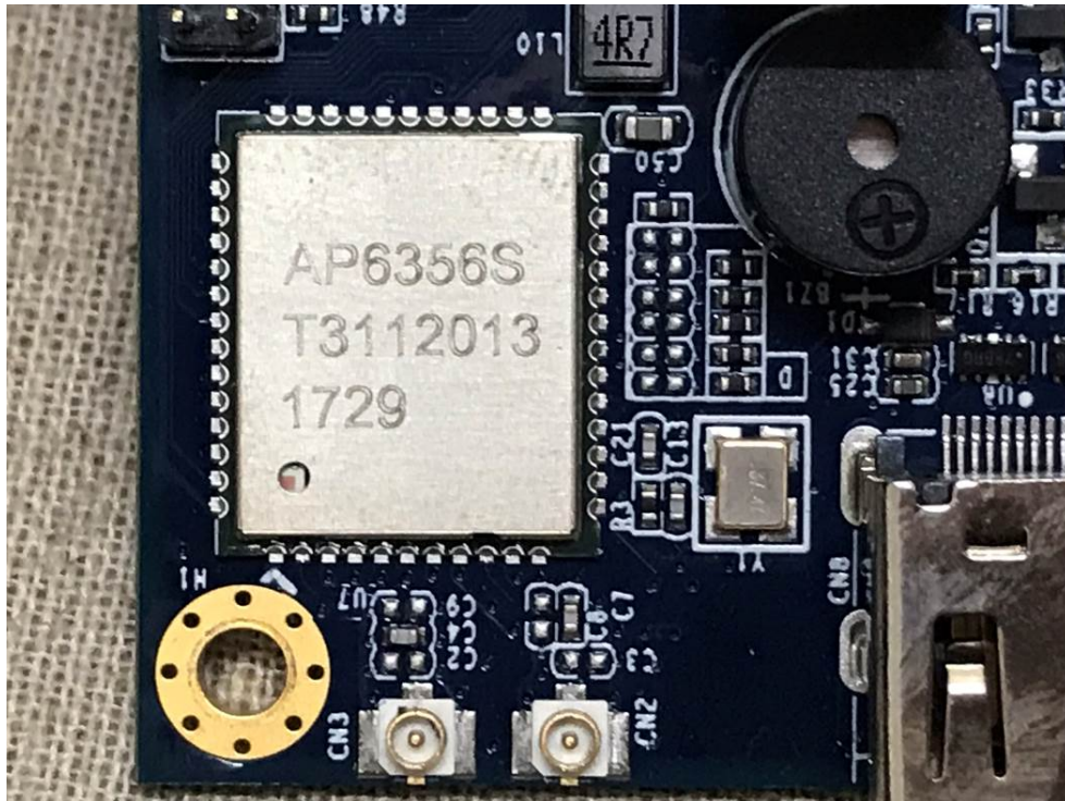
RF module
