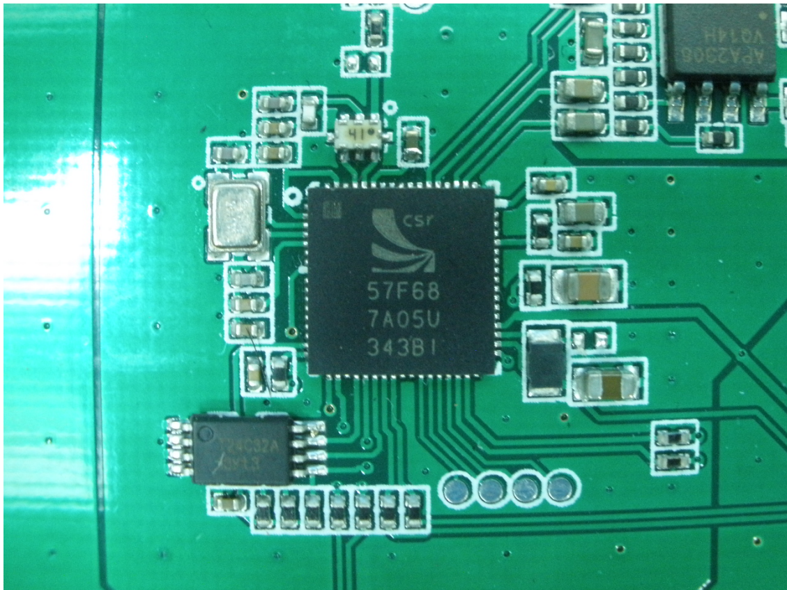
RF Module
