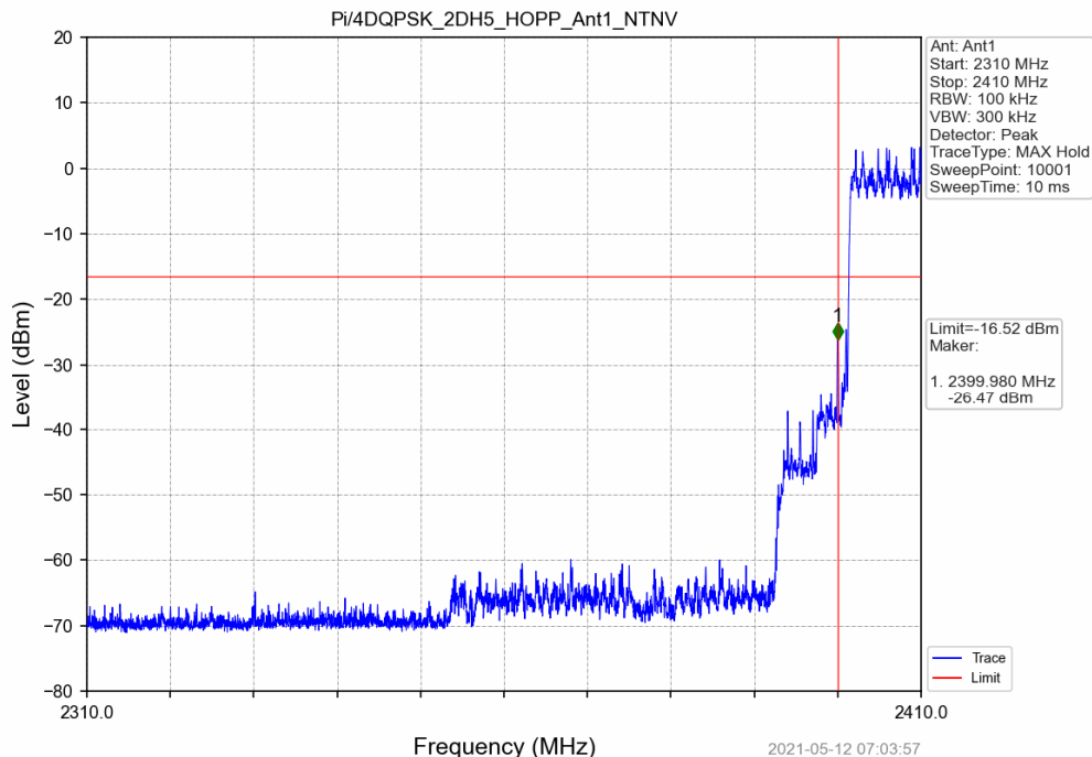
Pi/4DQPSK_2DH5_HOPP_Ant1_NTNV
