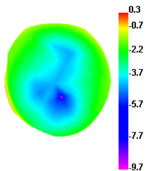
2500.000MHz E1
