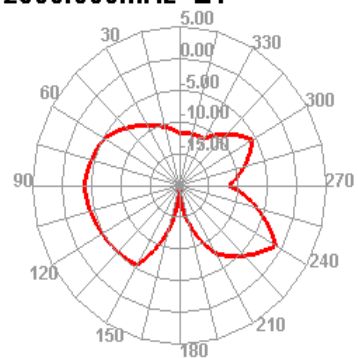
2500.000MHz E1
