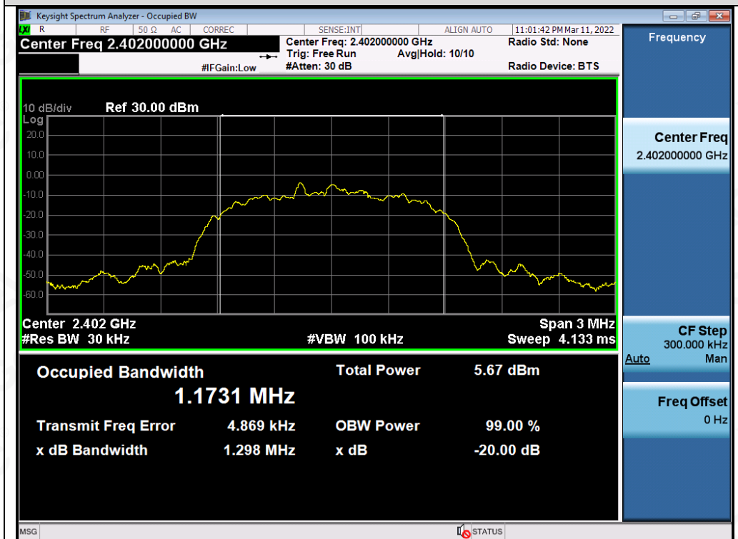
Test_Graph_EDR_ANT1_2402_3Mbps_OBW
