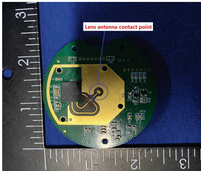
(14) EUT Photo
