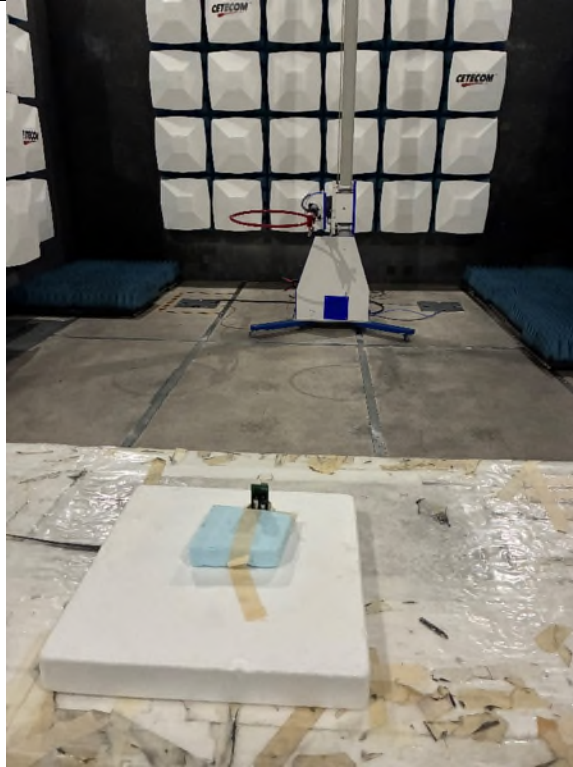
9kHz – 30MHz Rear
