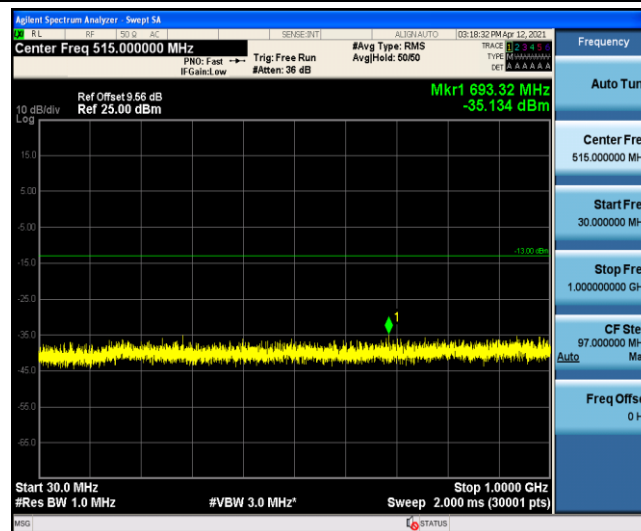
Band4-20MHz-QPSK-20050-1-0-Low-30-1000
