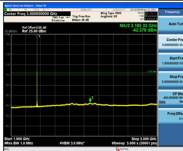
Band4-20MHz-QPSK-20050-1-0-Low-1000-5000
