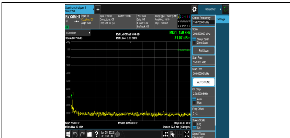
Band7-10MHz-QPSK-21400-1RB#0-Range2:0.15~30MHz
