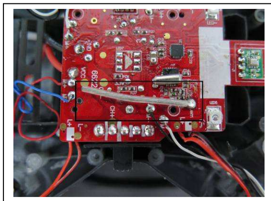
EUT antenna 1
