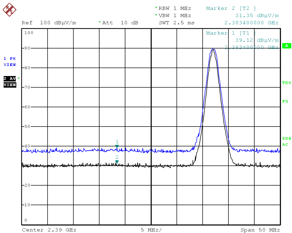
EDR(3DH5) Low(Vertical)
