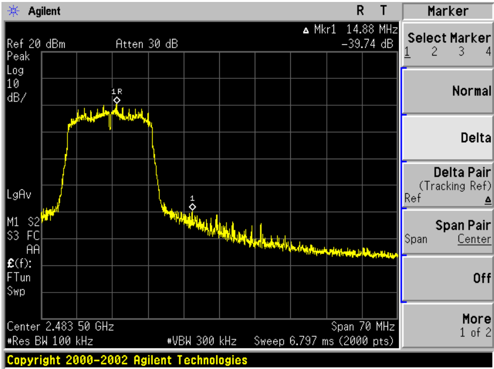
802.11g-CH11
