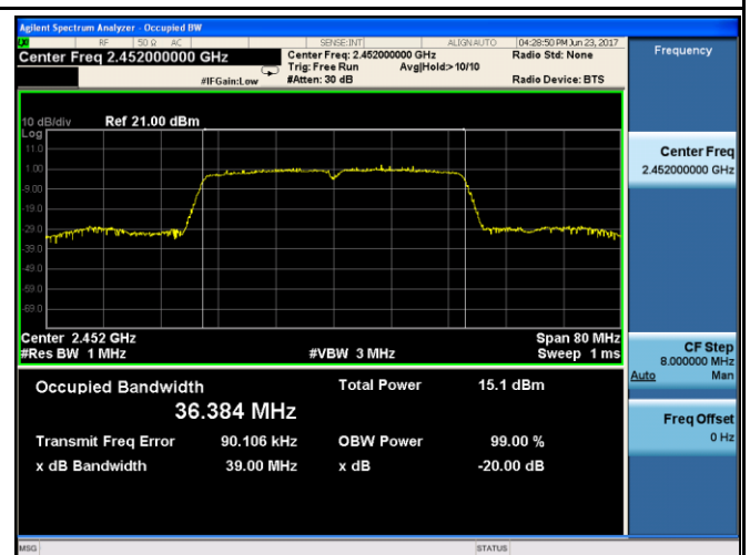
802.11n40 20dB Bandwidth - CH 9
