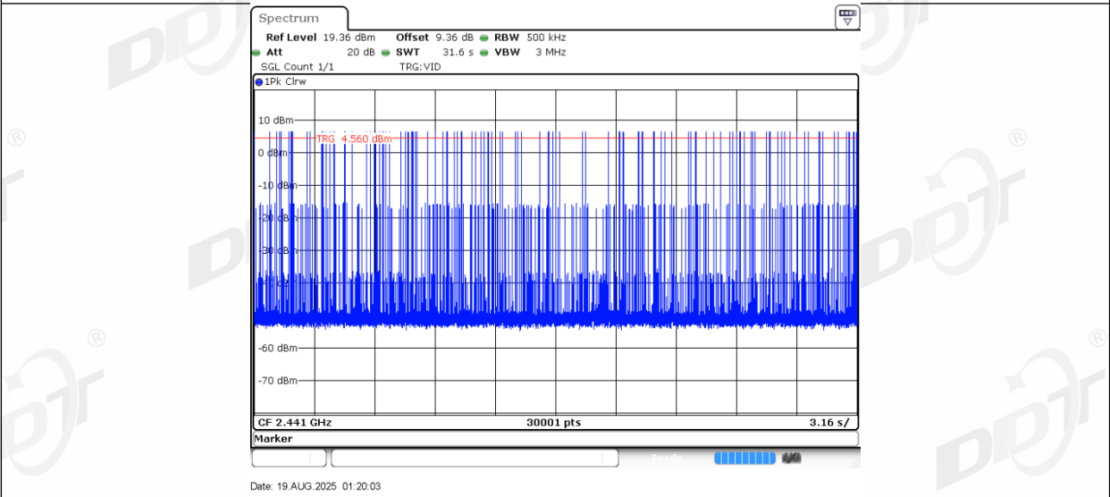
2DH1_Ant1_Hop
