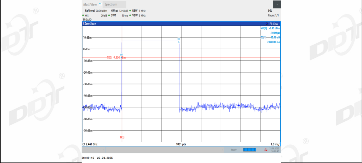
DH5_Ant2_Hop
