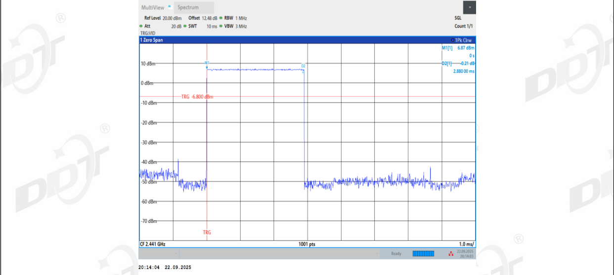
2DH5_Ant2_Hop
