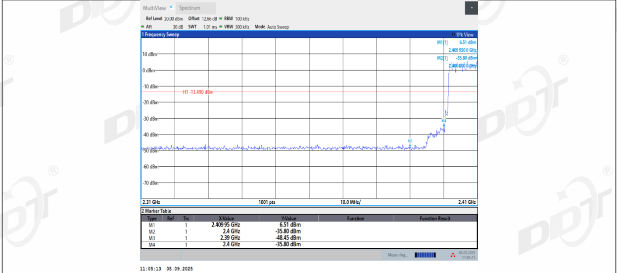
3DH5_Ant2_Low_Hop_2402
