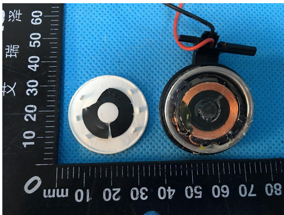
Internal Photos M/N: PS-AIO-8K-A
