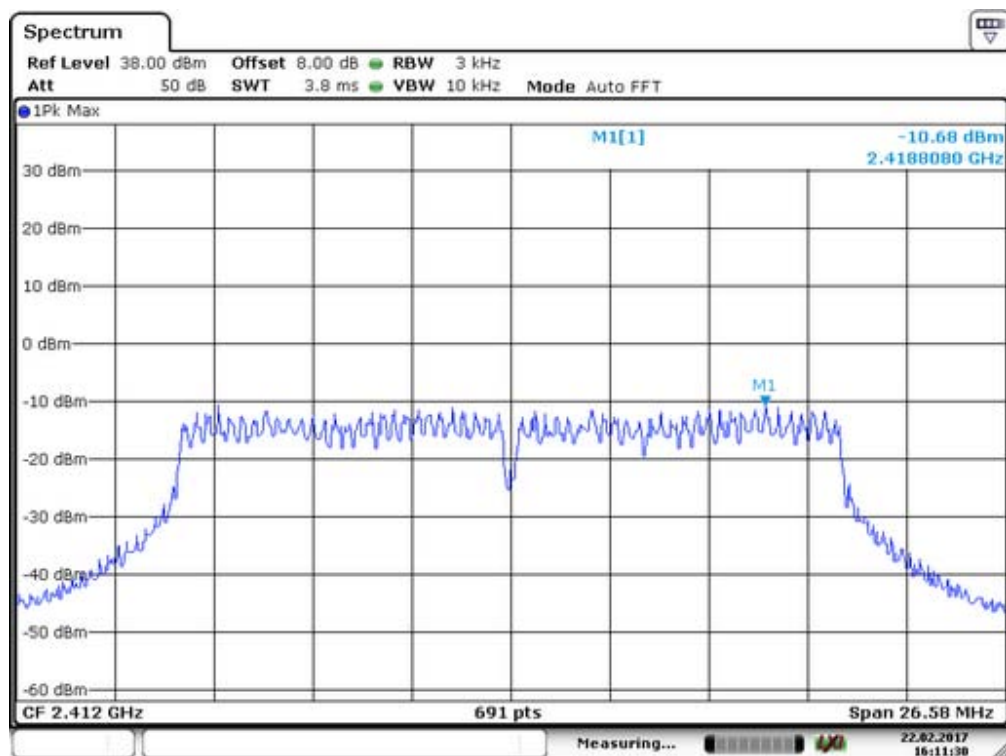
Ant1
