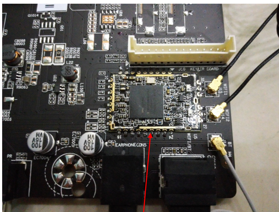
BT+WIFI Module
