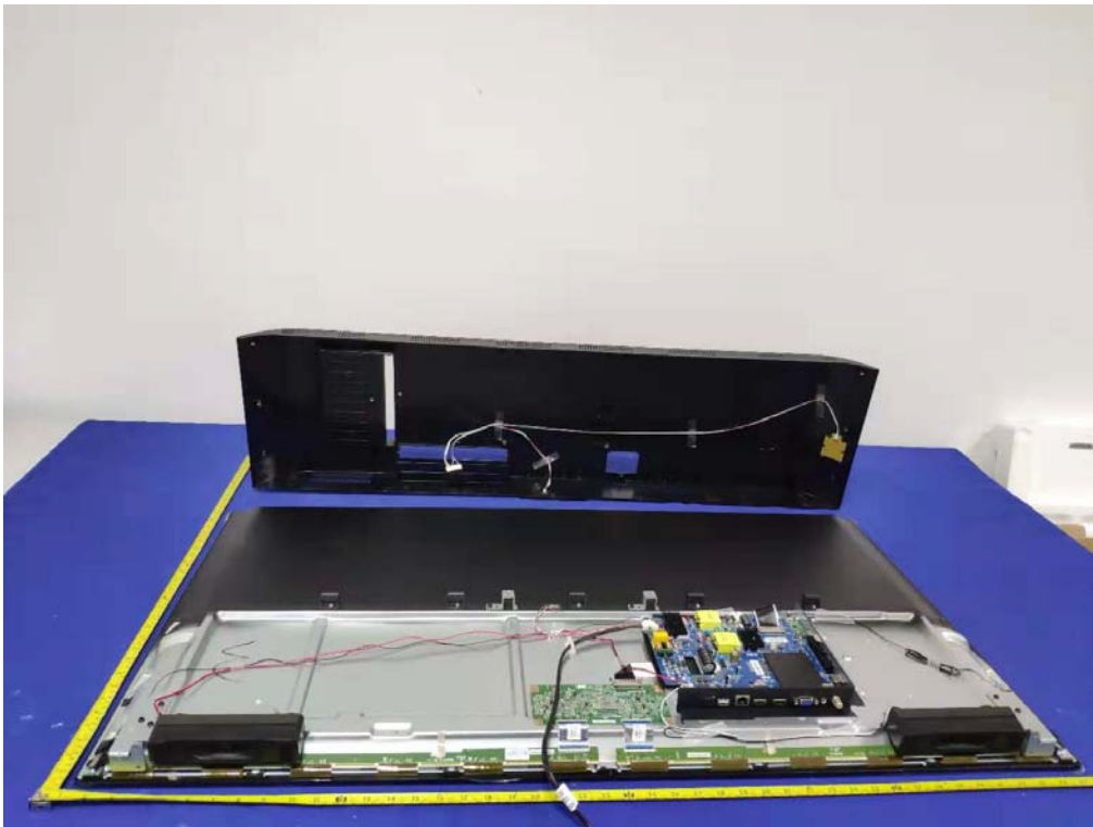
Internal photos M/N:WE50UE4008
