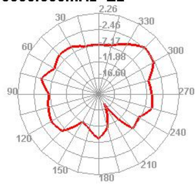
5850.000MHz E2
