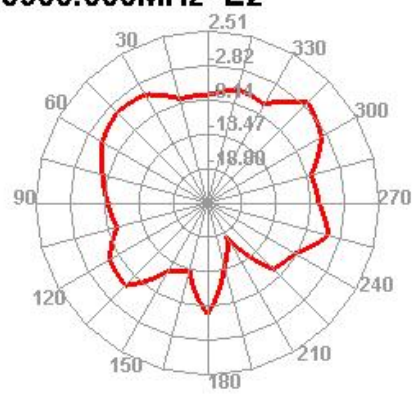
5900.000MHz E2
