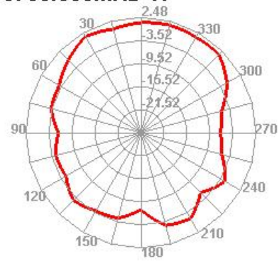
5700.000MHz H
