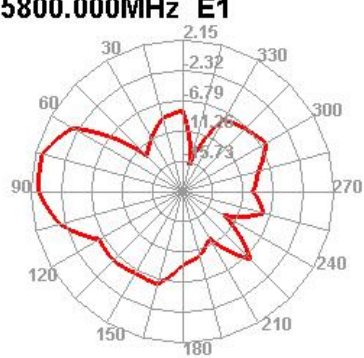
5800.000MHz E1
