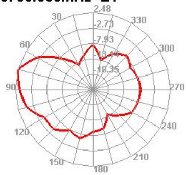
5700.000MHz E1
