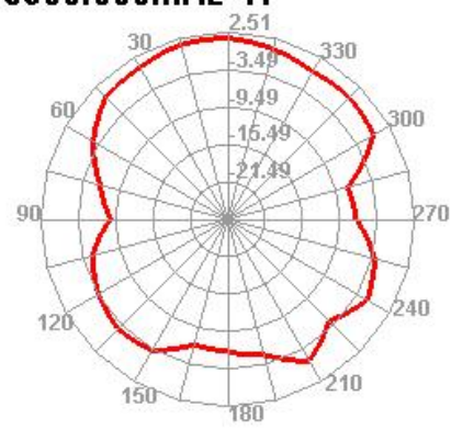
5900.000MHz H
