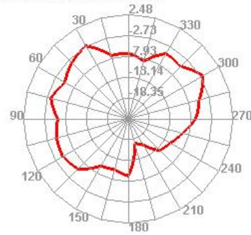
5700.000MHz E2
