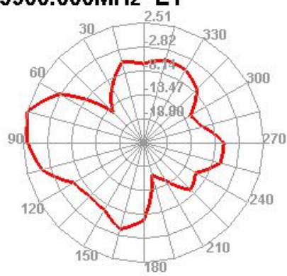
5900.000MHz E1
