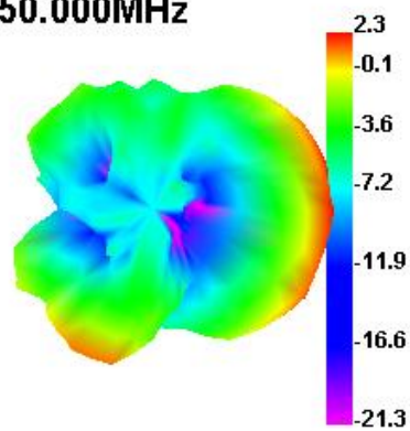
5850.000MHz
