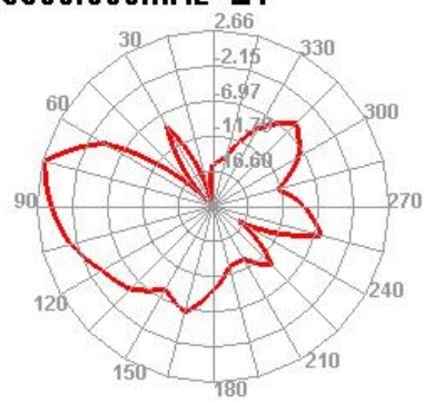
5500.000MHz E1
