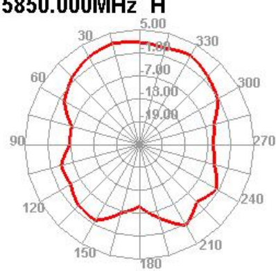
5850.000MHz H
