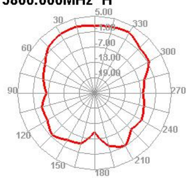
5800.000MHz H
