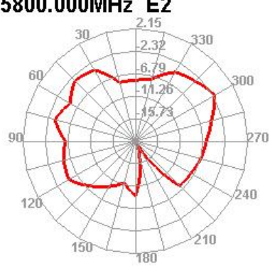
5800.000MHz E2
