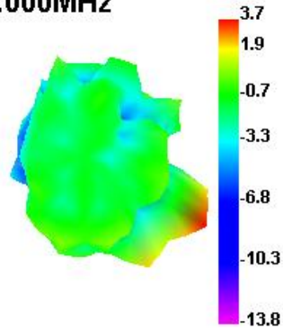
2450.000MHz E1
