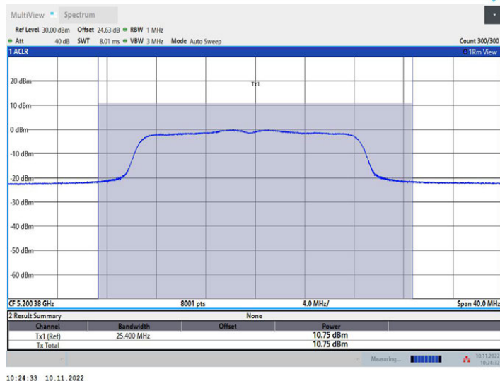
11N20MIMO_Ant1_5200
