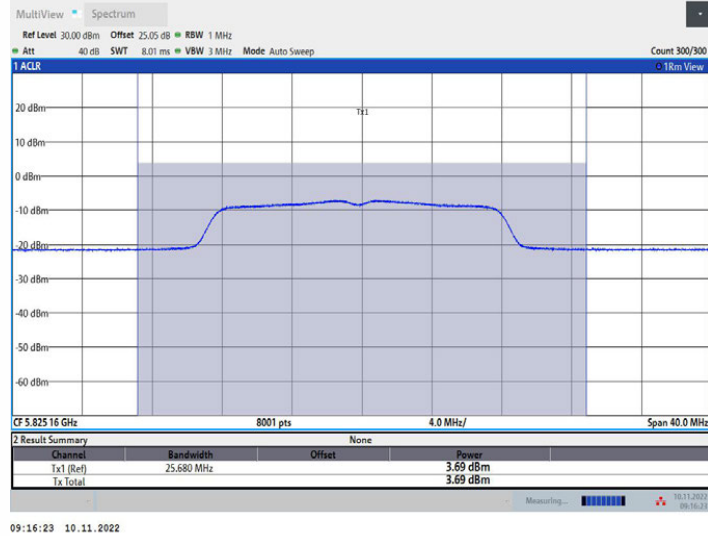
11A_Ant1_5825
