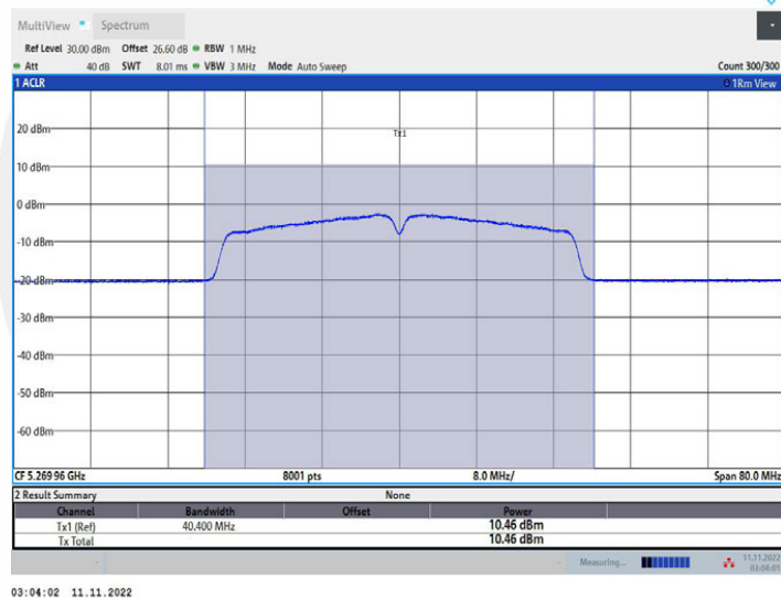
11AC40MIMO_Ant2_5270
