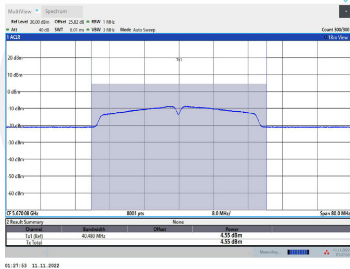
11N40MIMO_Ant2_5670
