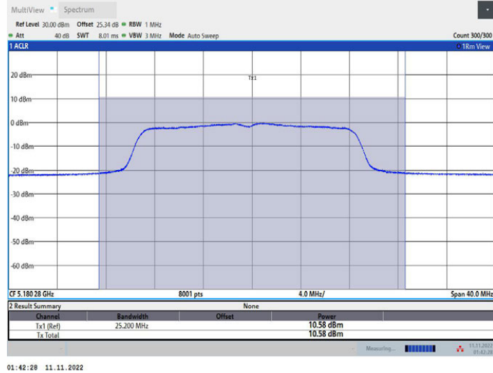
11AC20MIMO_Ant1_5180
