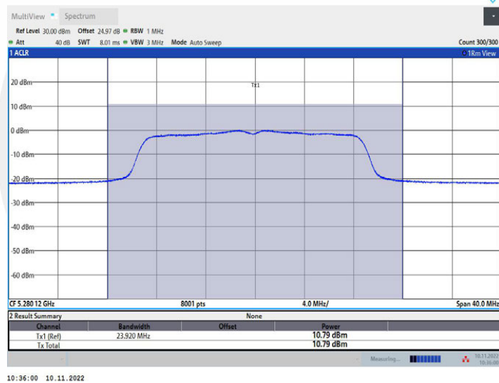
11N20MIMO_Ant2_5280
