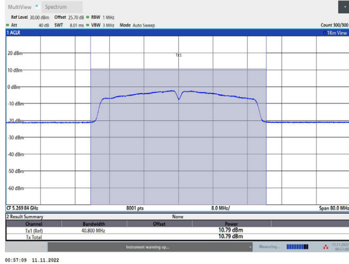
11N40MIMO_Ant1_5270
