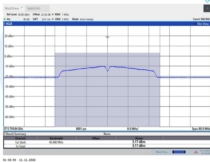
11N40MIMO_Ant2_5755
