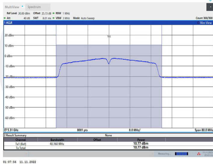
11N40MIMO_Ant2_5310
