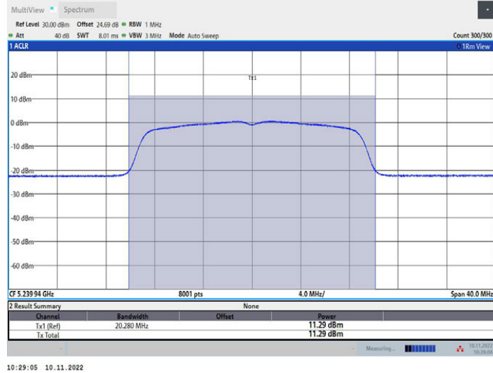
11N20MIMO_Ant1_5240
