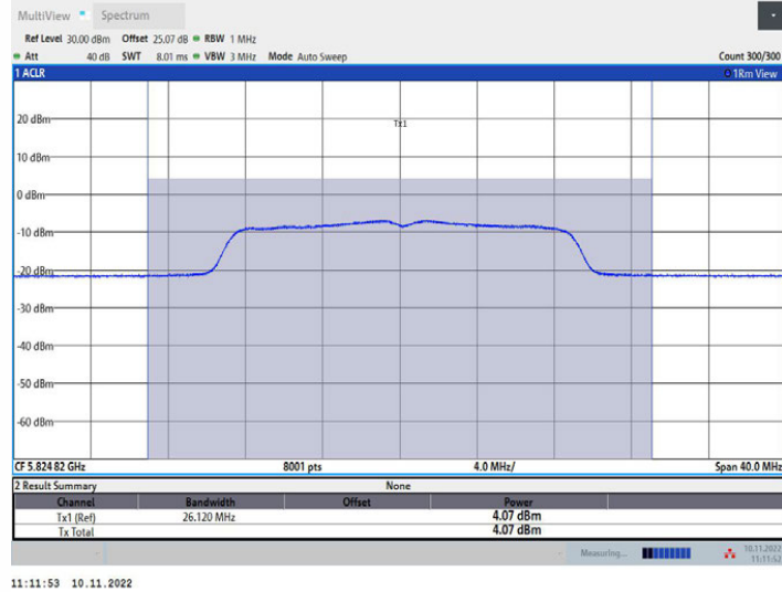
11N20MIMO_Ant1_5825
