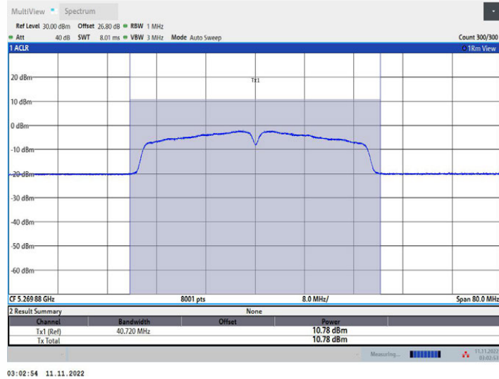
11AC40MIMO_Ant1_5270
