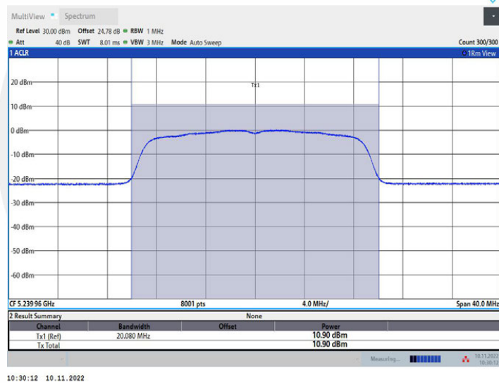
11N20MIMO_Ant2_5240
