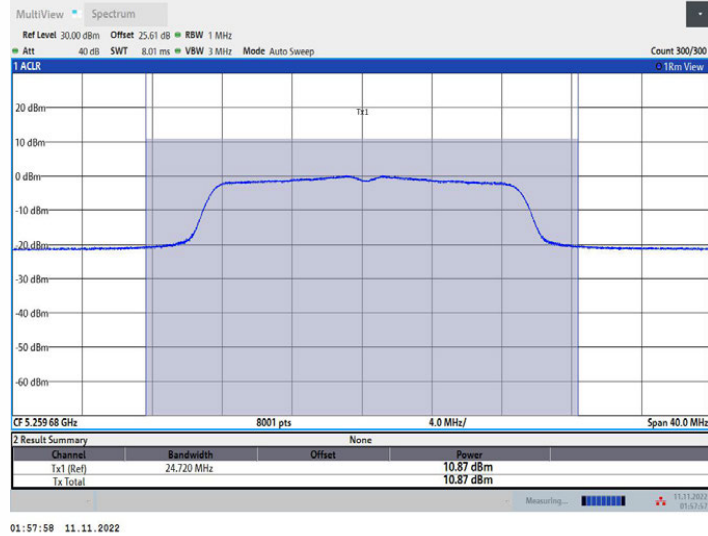
11AC20MIMO_Ant1_5260
