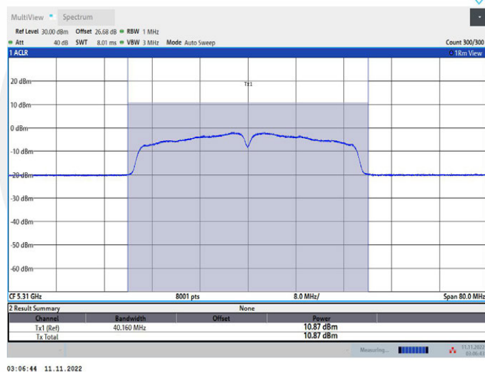
11AC40MIMO_Ant2_5310
