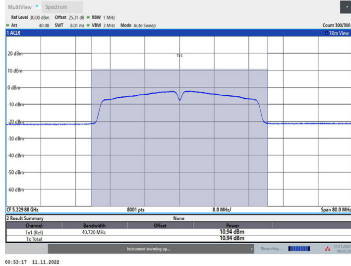
11N40MIMO_Ant1_5230
