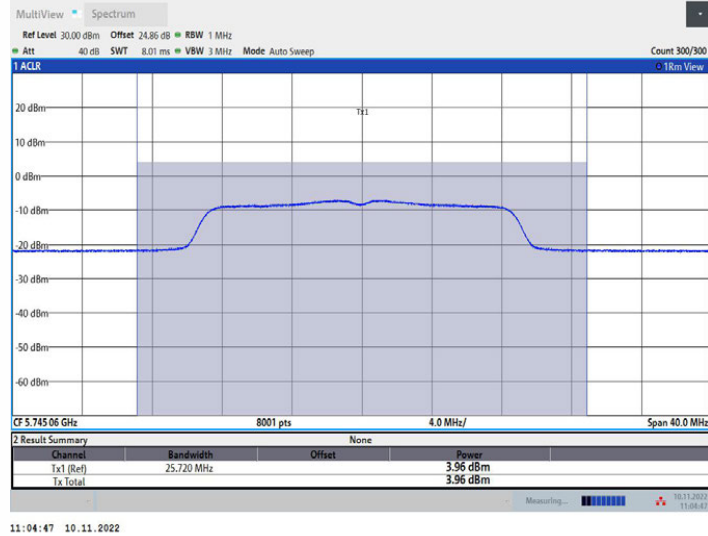
11N20MIMO_Ant1_5745
