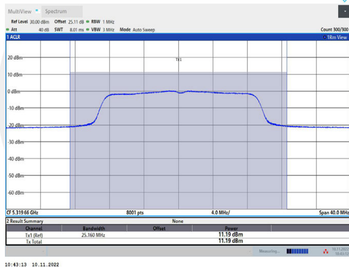
11N20MIMO_Ant2_5320
