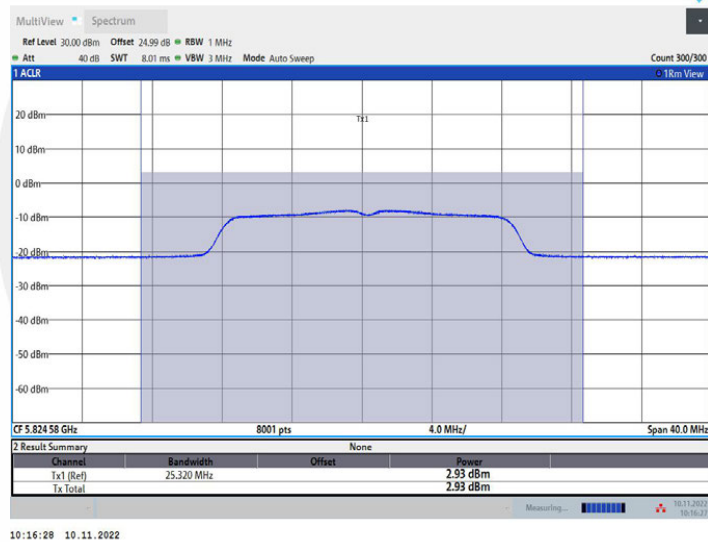
11A_Ant2_5825
