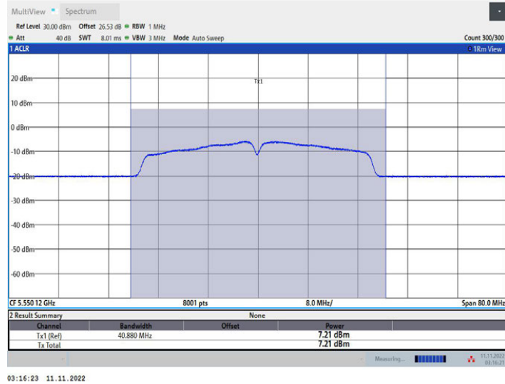
11AC40MIMO_Ant1_5550
