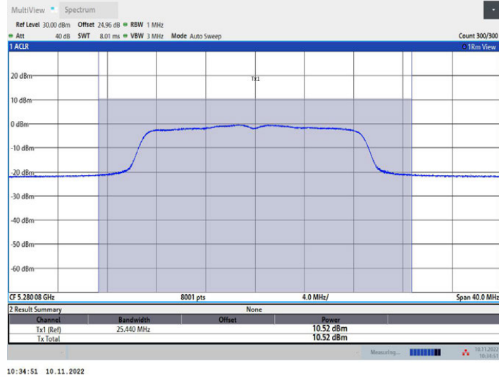
11N20MIMO_Ant1_5280
