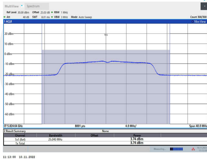
11N20MIMO_Ant2_5825
