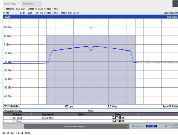
11N40MIMO_Ant1_5190
