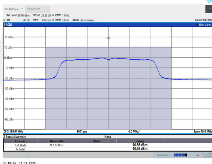
11AC20MIMO_Ant2_5200
