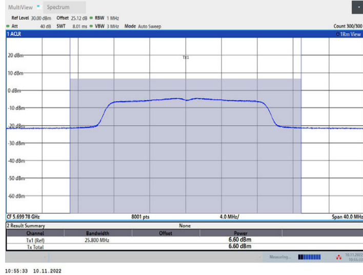
11N20MIMO_Ant1_5700
