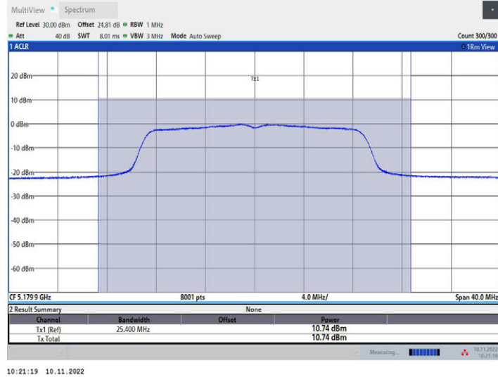
11N20MIMO_Ant1_5180
