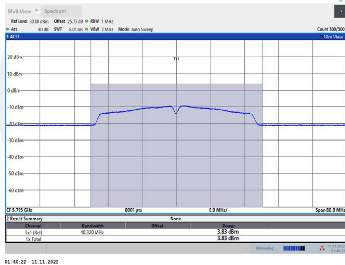
11N40MIMO_Ant2_5795
