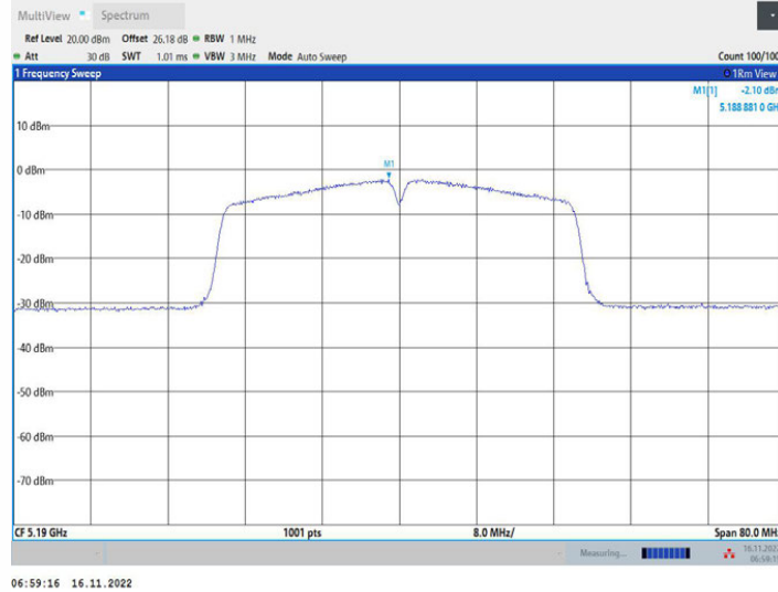
11AC40MIMO_Ant1_5190
