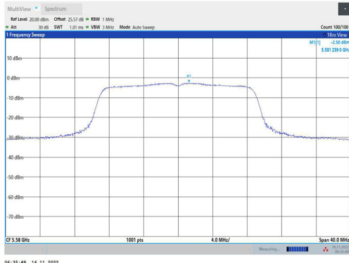
11AC20MIMO_Ant1_5580
