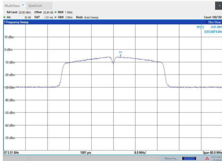
11AC40MIMO_Ant1_5510
