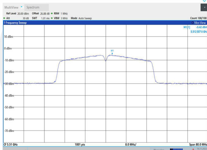
11AC40MIMO_Ant2_5510
