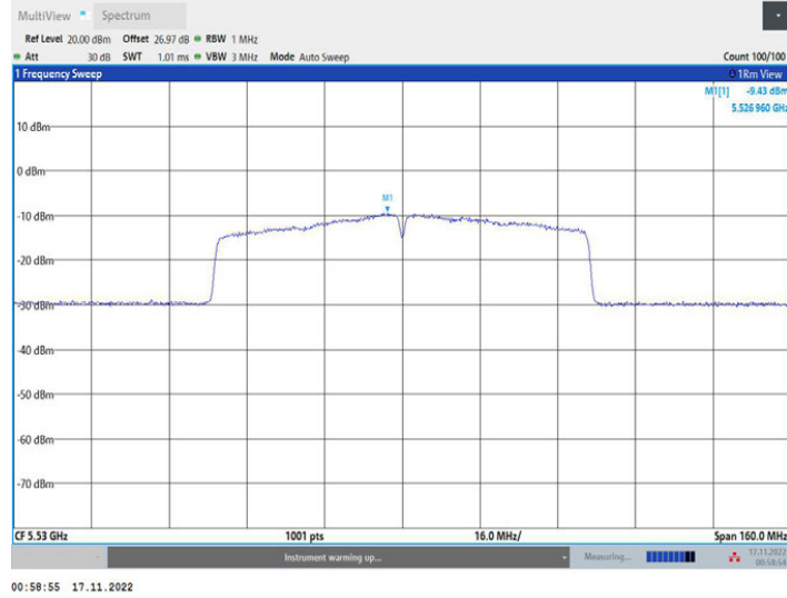
11AC80MIMO_Ant1_5530
