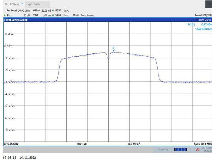
11AC40MIMO_Ant1_5550
