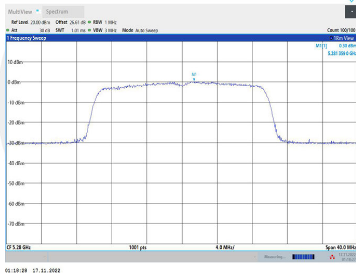
11AX20MIMO_Ant2_5280
