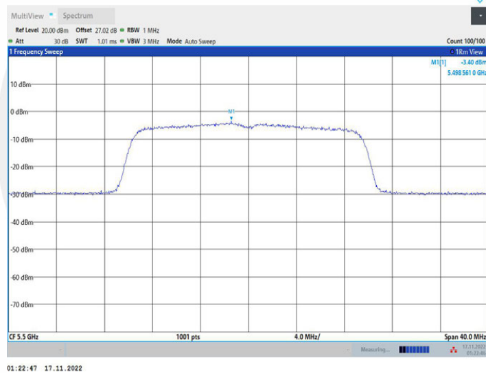
11AX20MIMO_Ant2_5500
