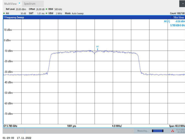
11AX20MIMO_Ant1_5785
