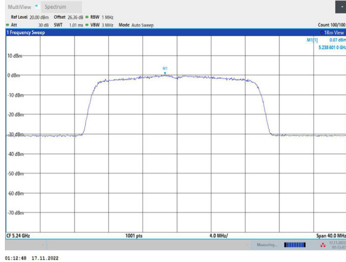
11AX20MIMO_Ant1_5240
