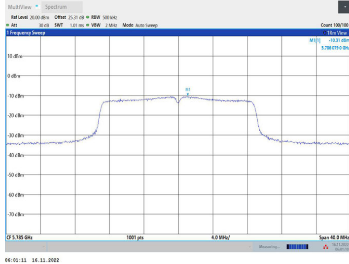
11N20MIMO_Ant1_5785
