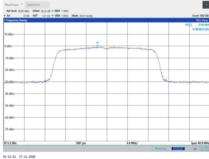
11AX20MIMO_Ant1_5200
