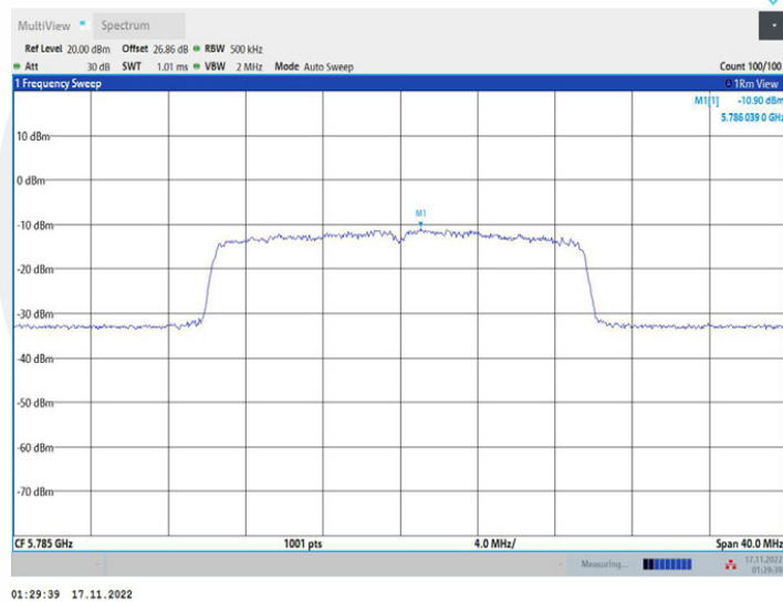
11AX20MIMO_Ant2_5785
