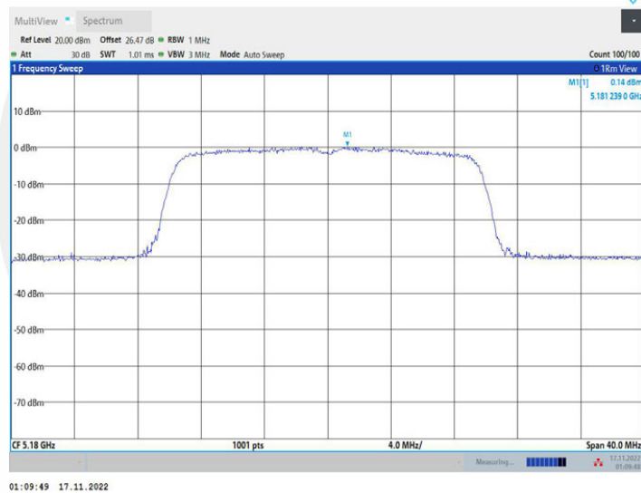
11AX20MIMO_Ant2_5180
