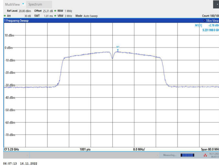
11N40MIMO_Ant1_5230
