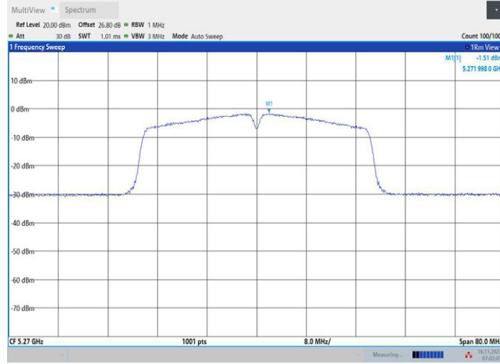
11AC40MIMO_Ant1_5270
