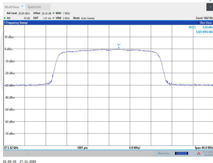
11AX20MIMO_Ant2_5320
