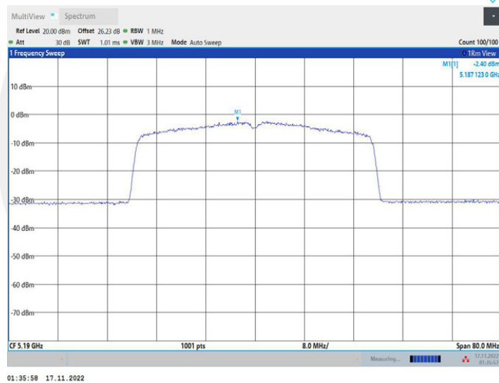
11AX40MIMO_Ant2_5190
