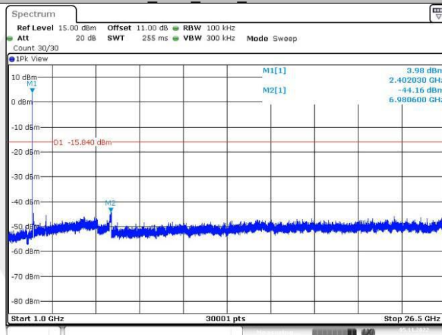
DH5_Ant1_2402_1000~26500
