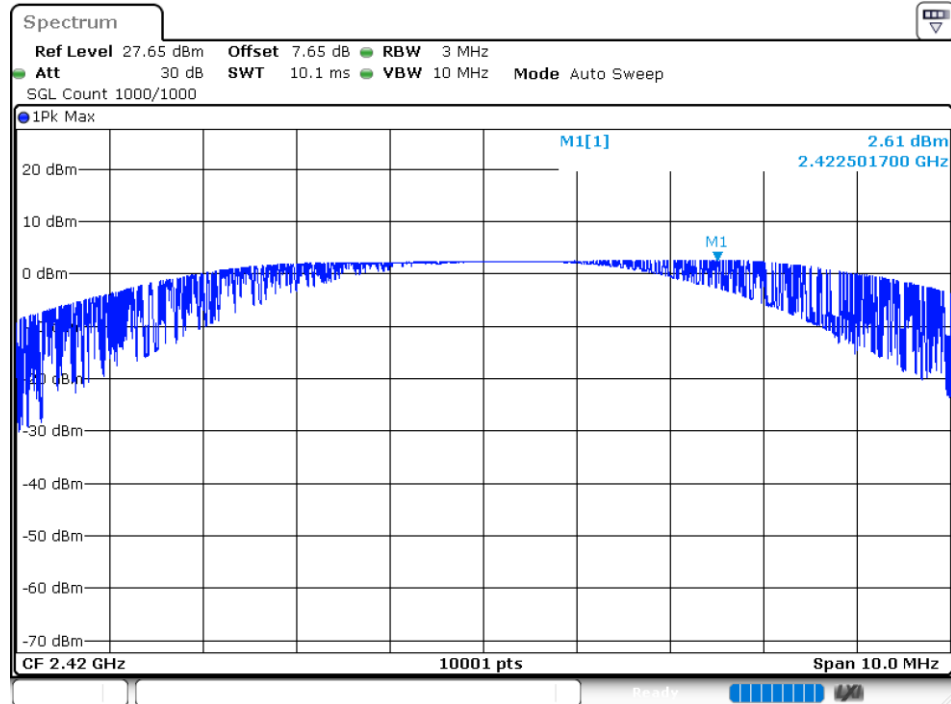
Power NVNT BLE 2420MHz Ant1
