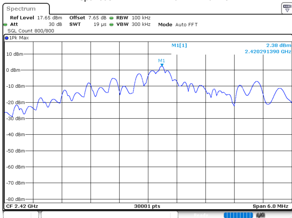
Tx. Spurious NVNT BLE 2420MHz Ant1 Ref
