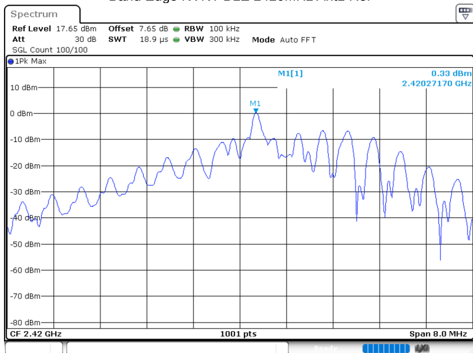
Band Edge NVNT BLE 2420MHz Ant1 Ref
