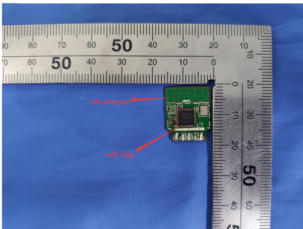
WI-FI module
