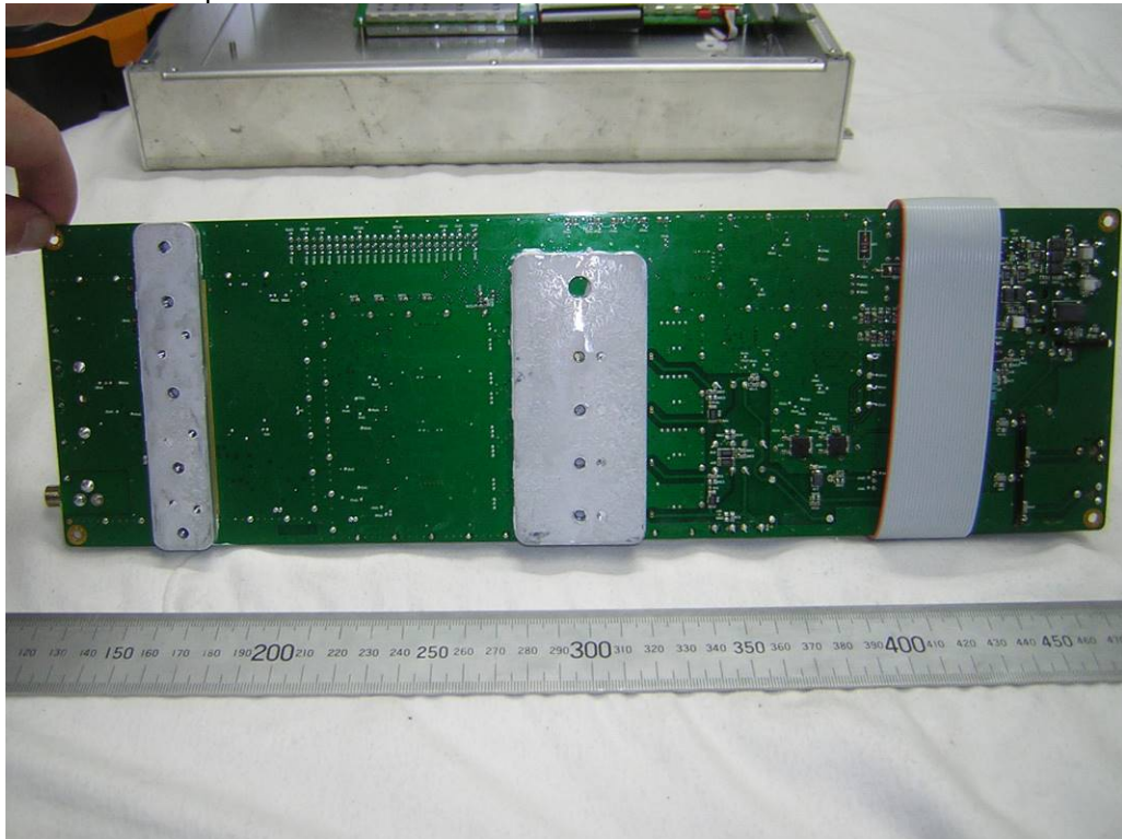
PCB Mars ATR Diplexer
