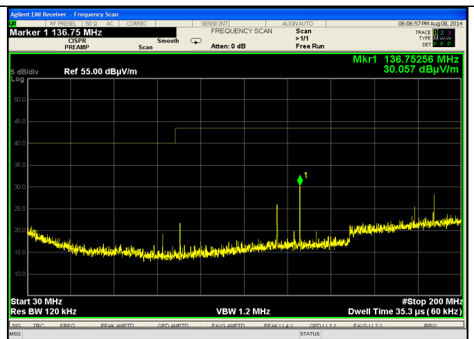
30-200 MHz Horizontal
