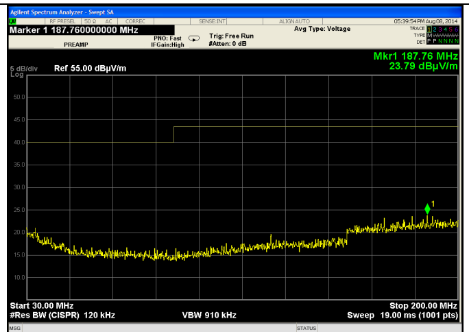
30-200 MHz Horizontal
