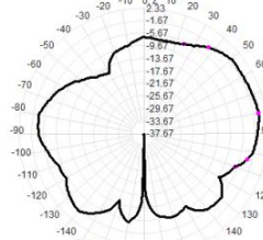
6600.0MHz Total(E2-YZ). Max= -0.34dBi
