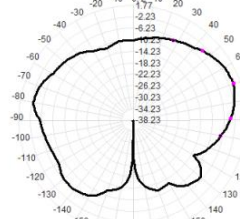
6300.0MHz Total(E2-YZ). Max= 0.88dBi
