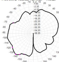
7100.0MHz Total(E2-YZ), Max= -1.05dBi
