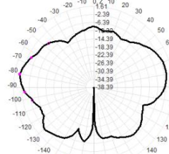
6400.0MHz Total(E2-YZ). Max= -1.04dBi
