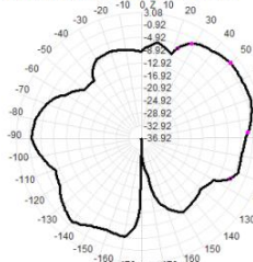
6900.0MHz Total(E2-YZ), Max= 0.42dBi
