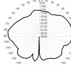
6500.0MHz Total(E2-YZ). Max= 0.18dBi
