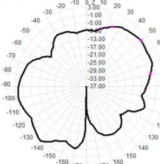
7000.0MHz Total(E2-YZ), Max= -0.83dBi
