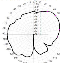
7200.0MHz Total(E2-YZ), Max= 0.53dBi
