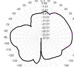
6700.0MHz Total(E2-YZ). Max= -1.86dBi
