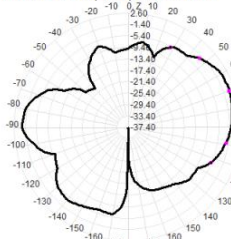
6800.0MHz Total(E2-YZ), Max= 0.38dBi
