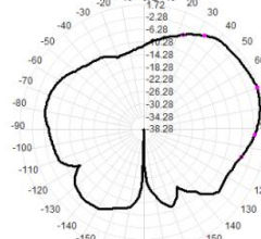
6200.0MHz Total(E2-YZ). Max= 0.74dBi
