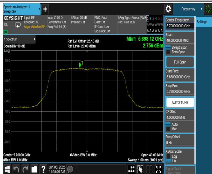
11AX20MIMO_Ant2_5700
