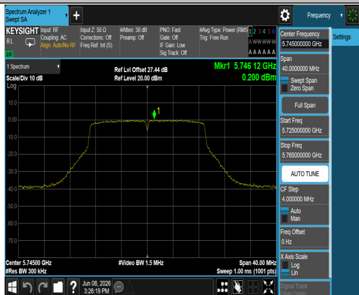
11AC20MIMO_Ant1_5745
