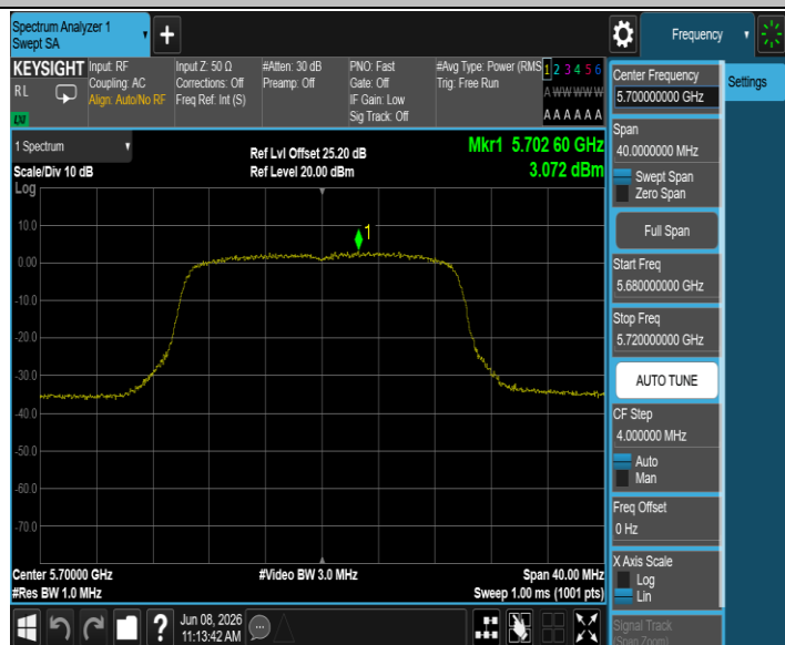
11AX20MIMO_Ant2_5700
