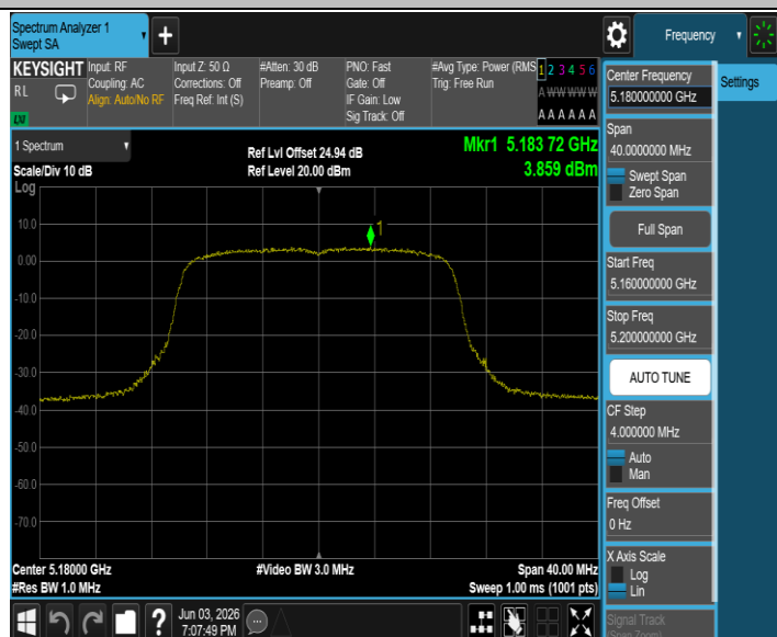
11BE20MIMO_Ant2_5180
