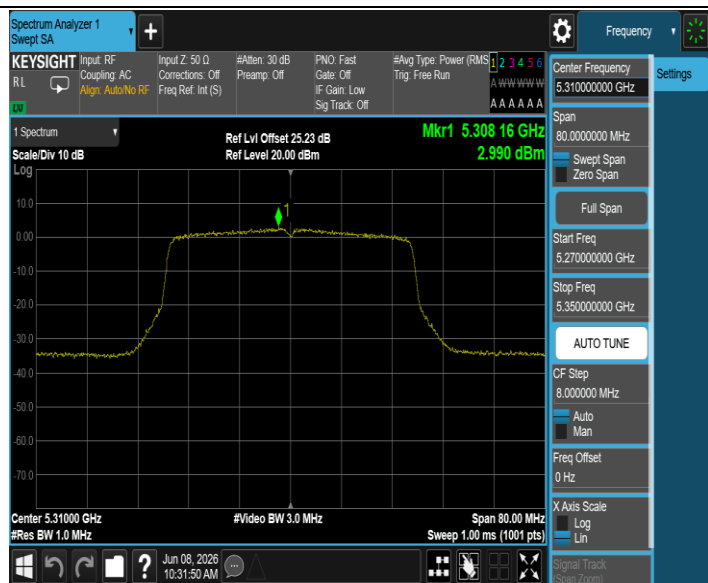
11AX40MIMO_Ant2_5310
