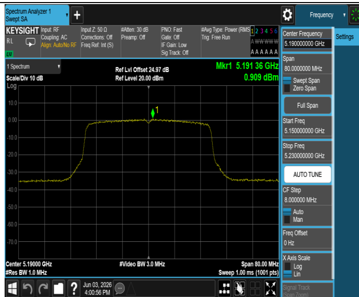
11BE40MIMO_Ant2_5190
