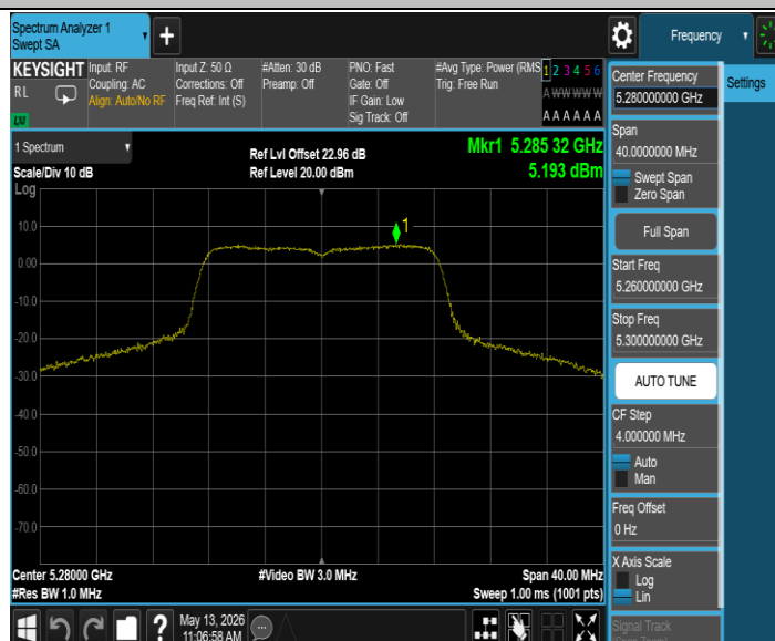
11A_Ant3_5280
