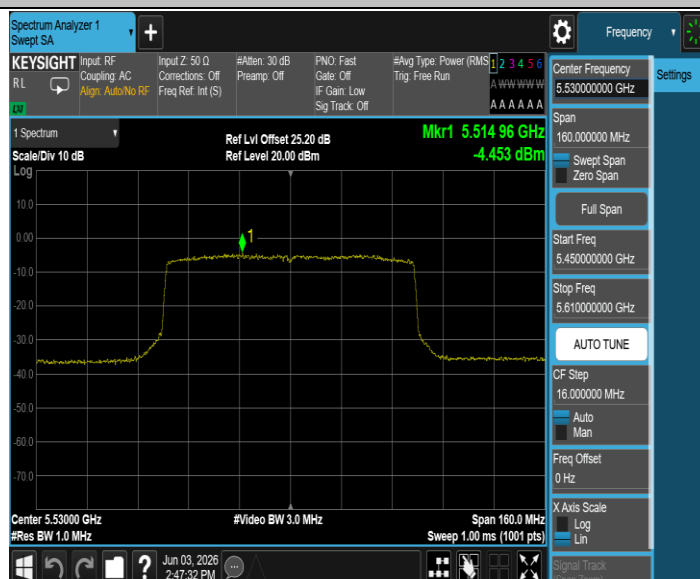
11BE80MIMO_Ant1_5530
