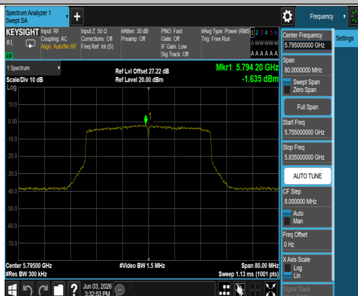
11BE40MIMO_Ant2_5795
