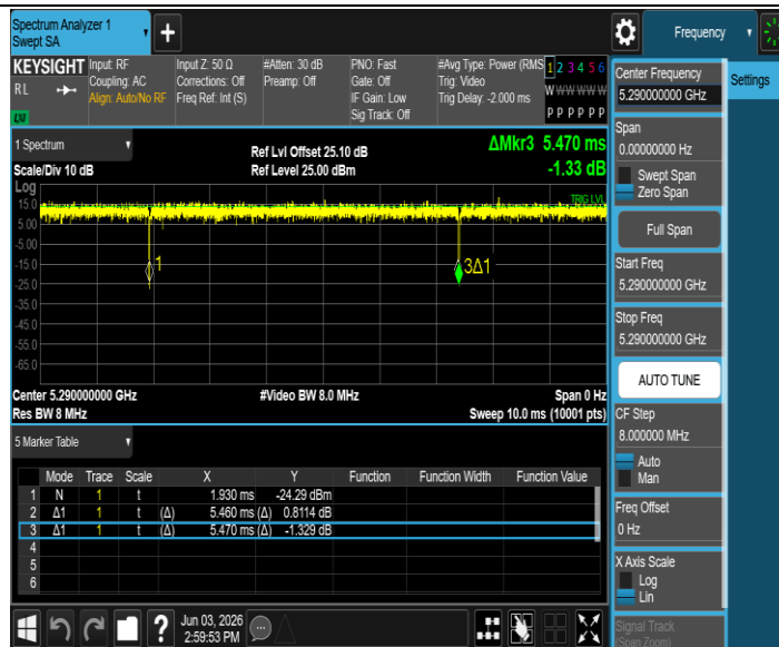
11BE80MIMO_Ant2_5290
