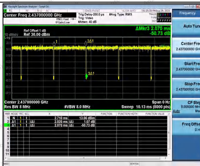
11G_Ant2_2437
