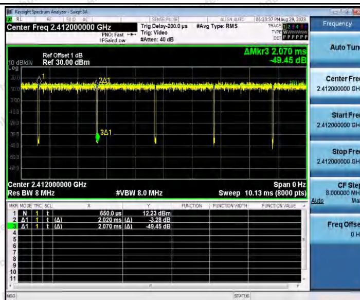
11G_Ant2_2412
