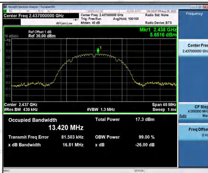
11B_Ant2_2437
