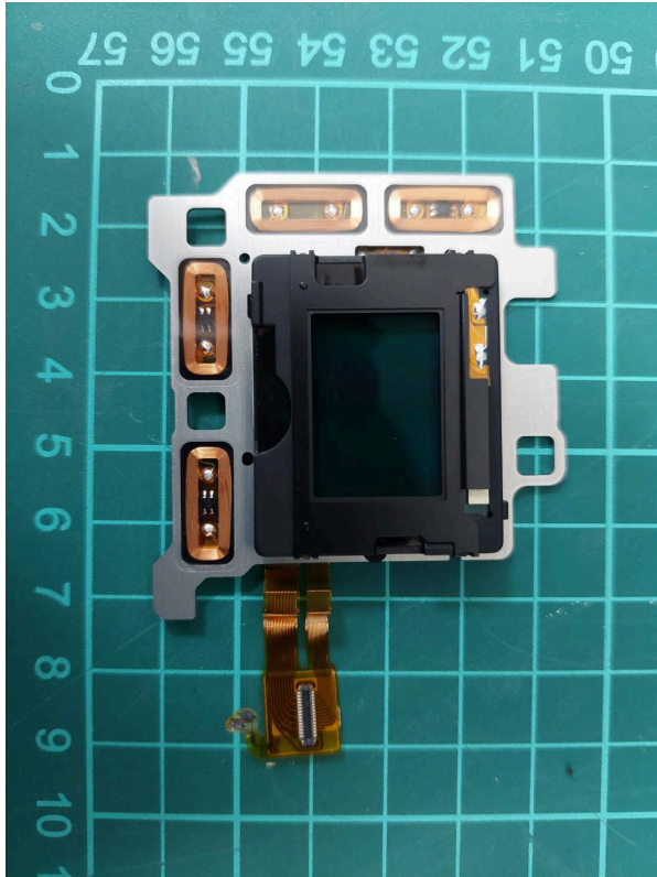
(15) EUT Photo
