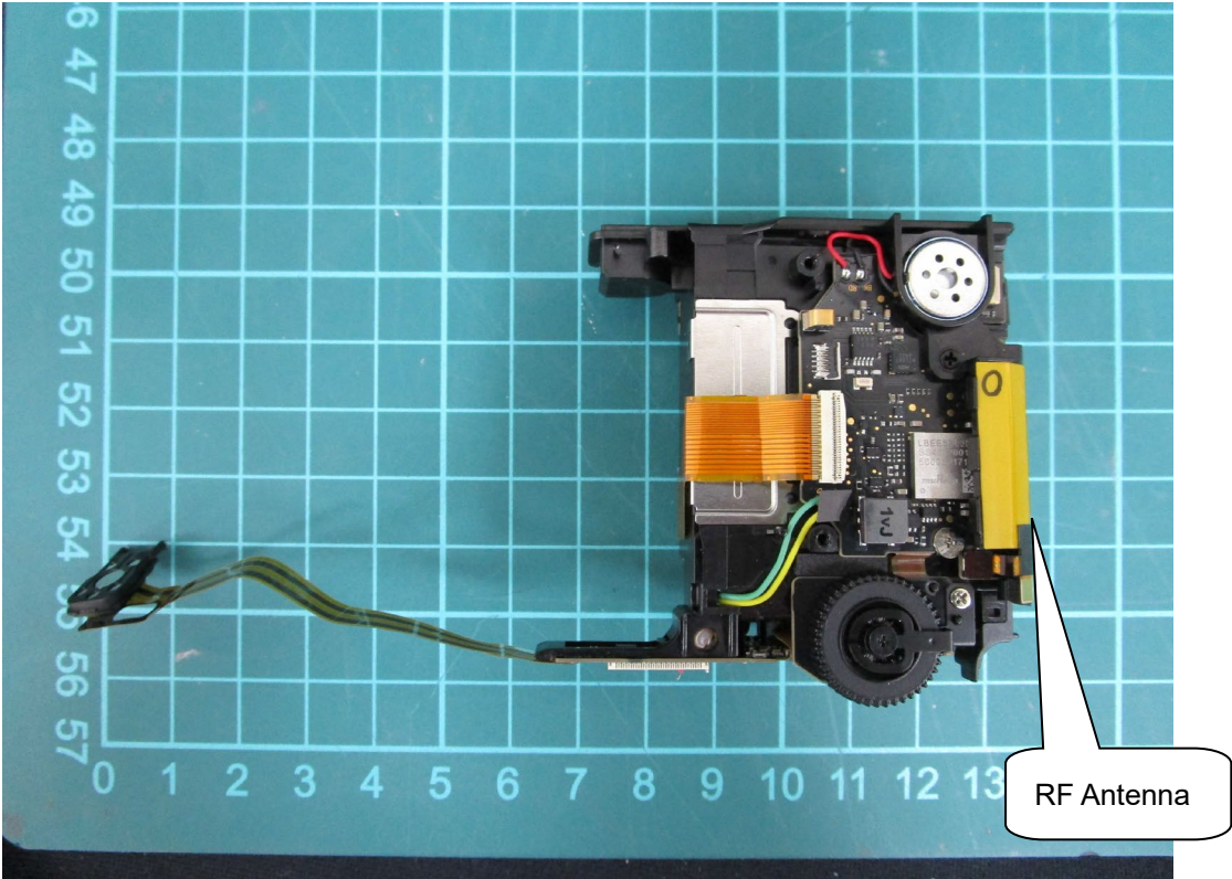
(21) EUT Photo
