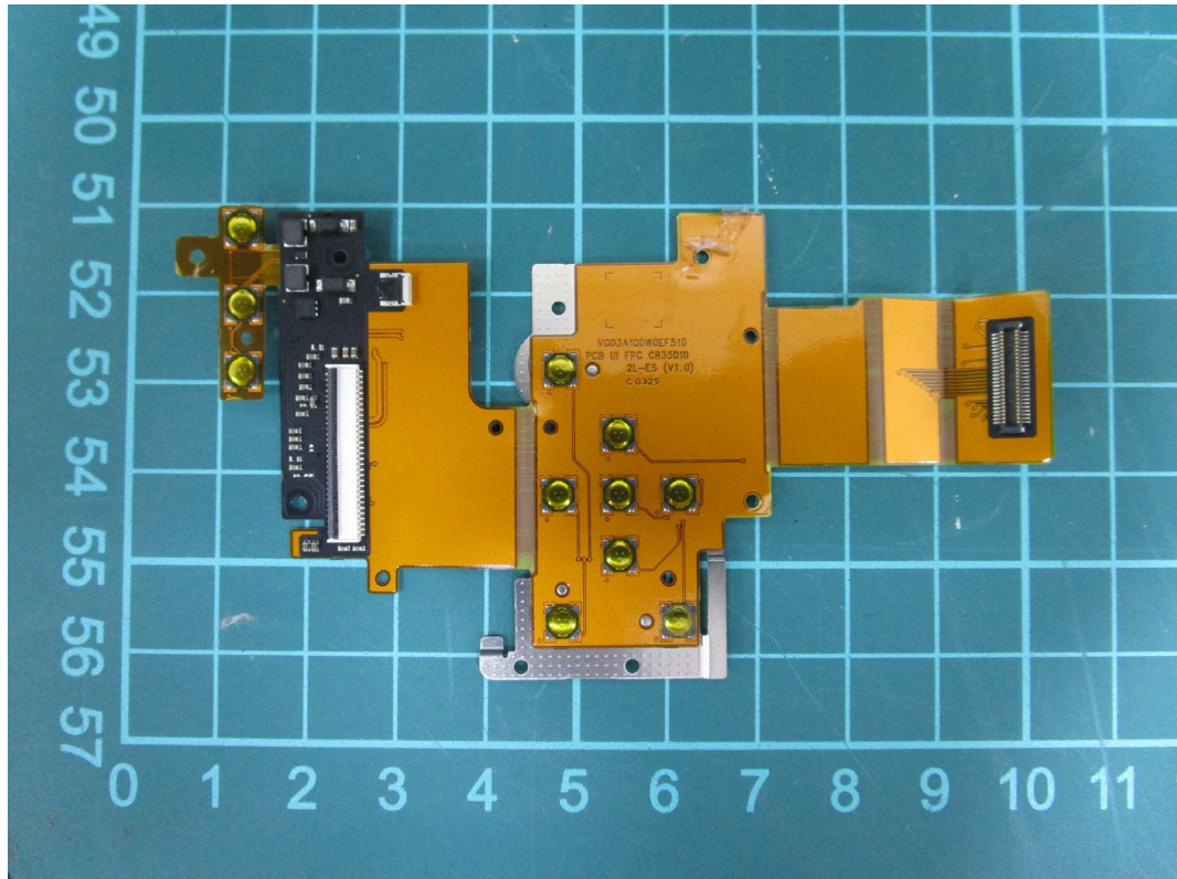
(5) EUT Photo
