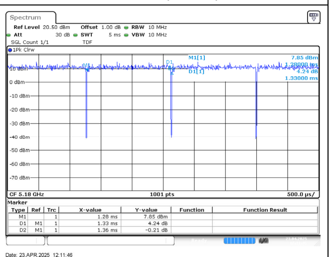
802.11ac (20 MHz)
