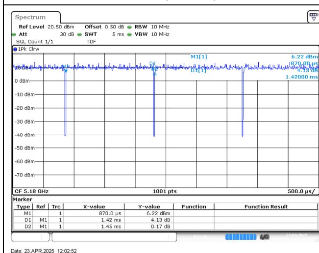
802.11a (20 MHz)
