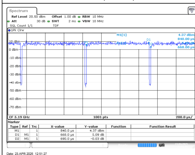
802.11ac (40 MHz)
