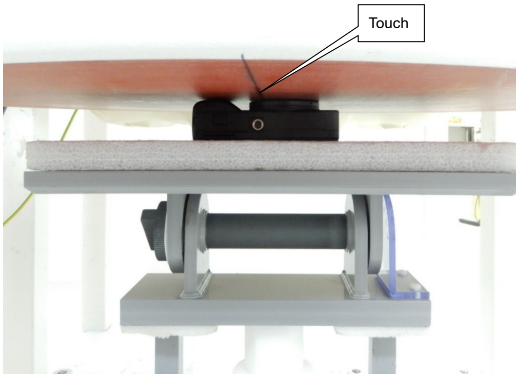
EUT Left-side
