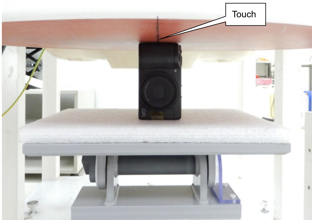
EUT Left-side
