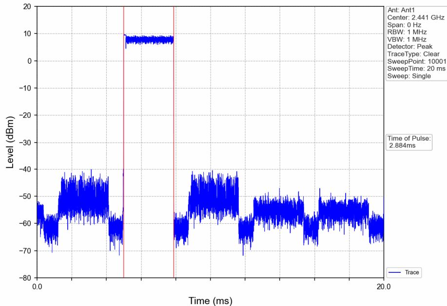
8DPSK_3DH5_HOPP_Ant1_NTNV
