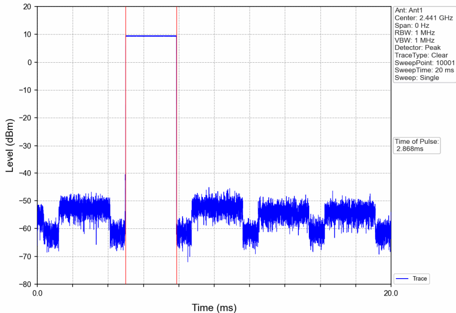
GFSK_DH5_HOPP_Ant1_NTNV
