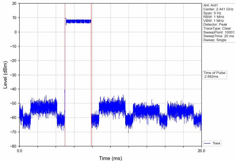
Pi/4DQPSK_2DH5_HOPP_Ant1_NTNV
