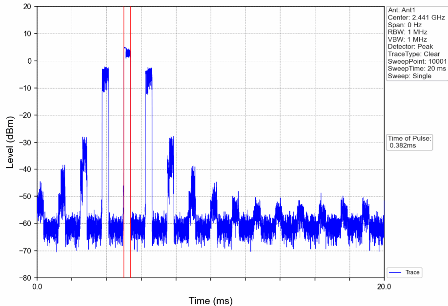
8DPSK_3DH1_HOPP_Ant1_NTNV
