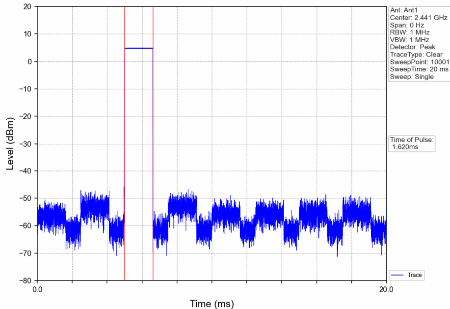
GFSK_DH3_HOPP_Ant1_NTNV
